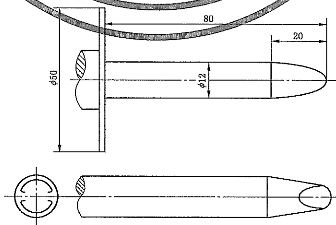
图 10 刚性试验指
