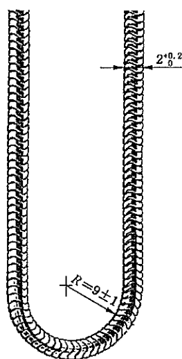
图 11 试验链
