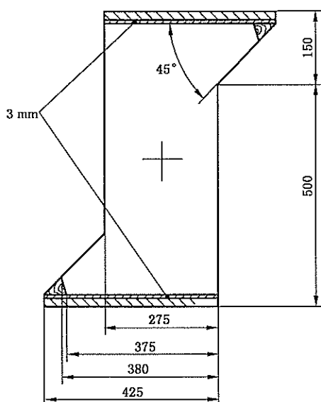
图 8 滚筒
