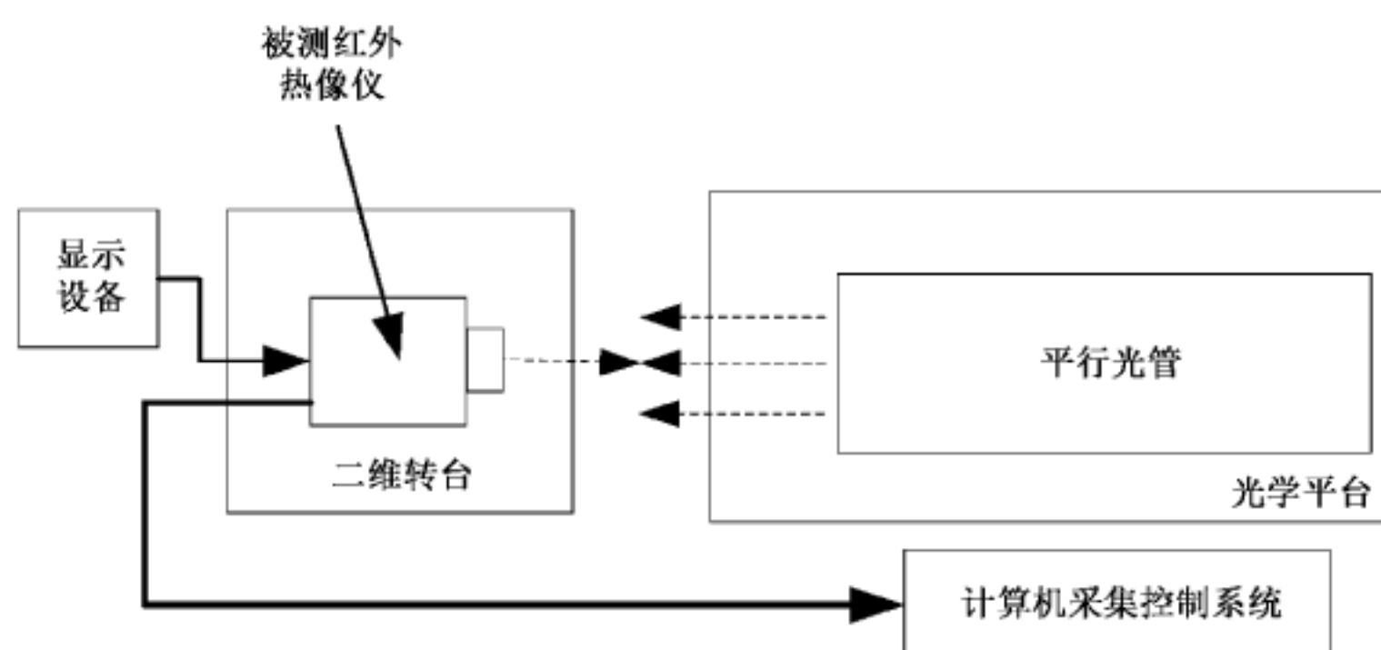
图3 热像仪置于二维转台示意图
