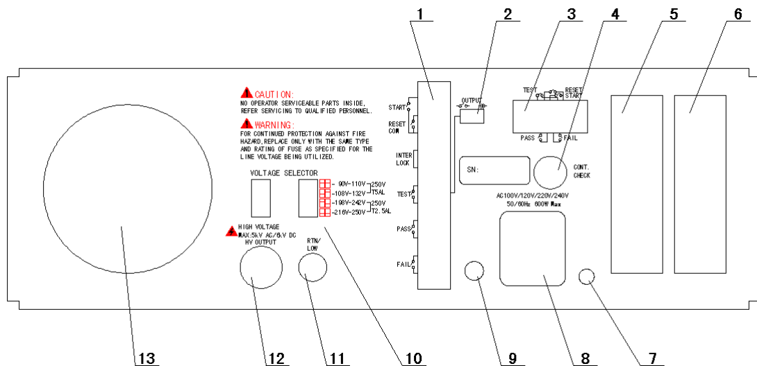
图 3-2 后面板说明
