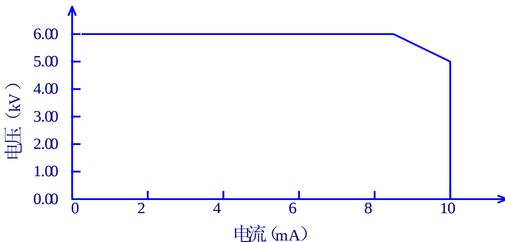
图 3-4 9058 直流电压输出范围
