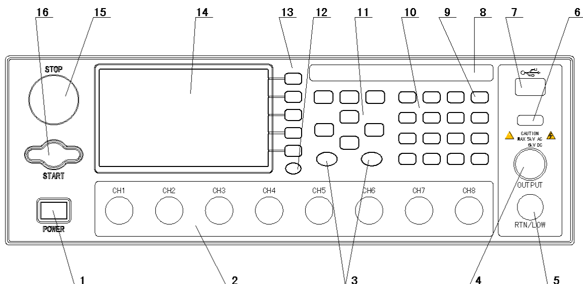
图 3-1 前面板说明
