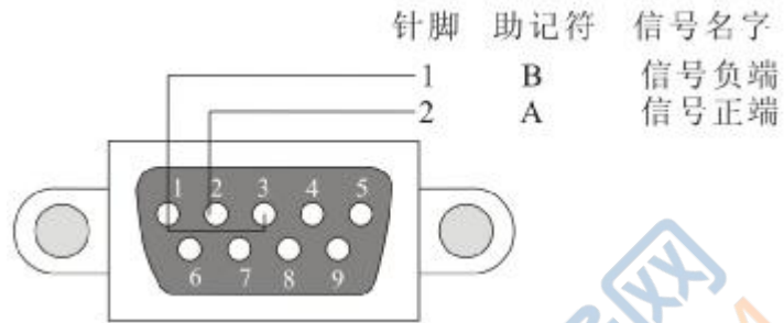
图 5.2.2 RS-485 接口
