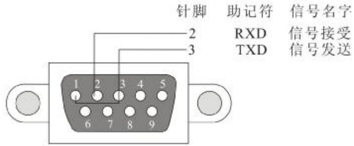
图 5.2.1 RS-232 接口
