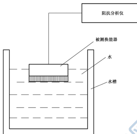
图 8 平面阵(或曲面阵)等效电阻测量原理图
