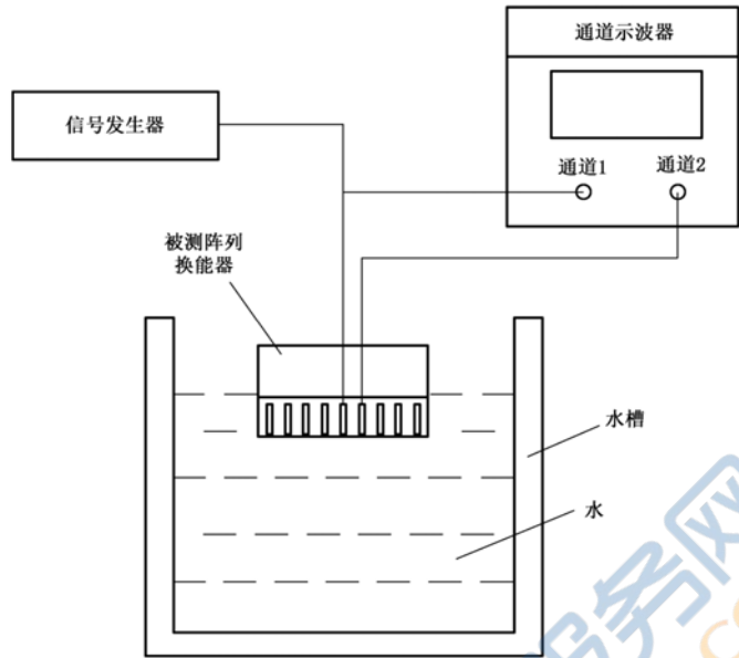
图 7 阵列换能器阵元互耦度测量原理图
