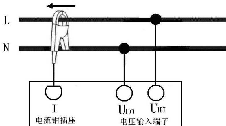
图 12 8700A 测量负载接线原理图
