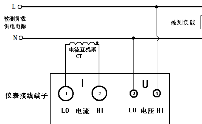
图7 8700A/B 测量负载接互感器原理图
