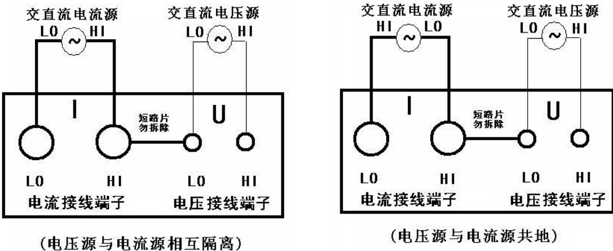
图 10 8700C 检定接线图
