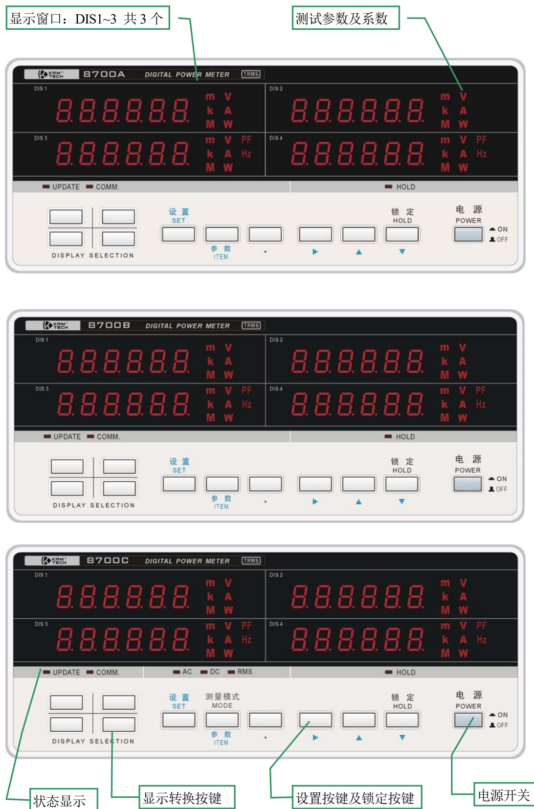
图 2 8700A/B/C 仪表前面板示意图
