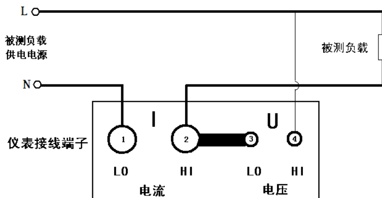
图6 8700A/B/C 仪表测量负载接线(不带互感器)原理图
