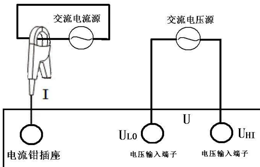
图 13 8700A（带电流钳）检定接线图
