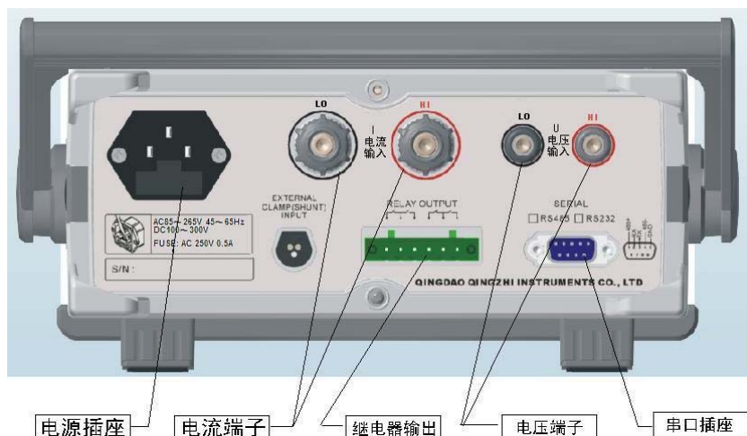
图4 8700A/B/C 后面板示意图
