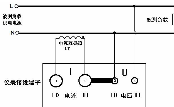
图8 8700C 测量负载接互感器原理图
