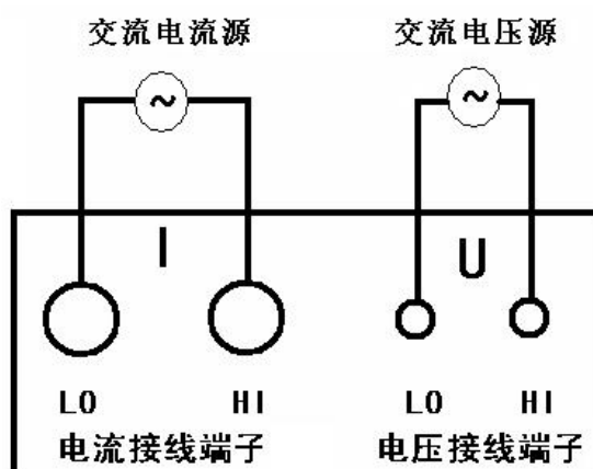
图9 8700A/B 检定接线图
