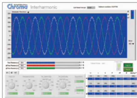
间谐波测试
