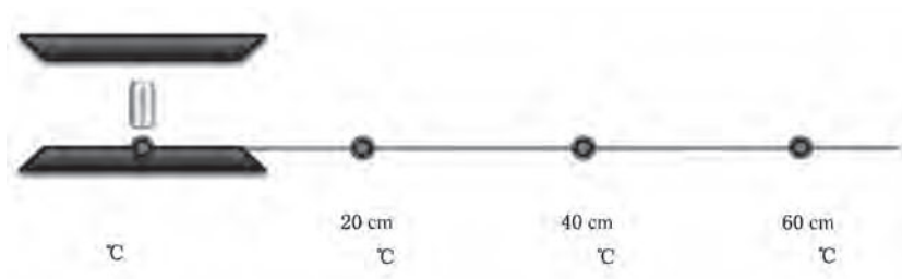
图 6 异物检测的温升试验和灼热试验图
