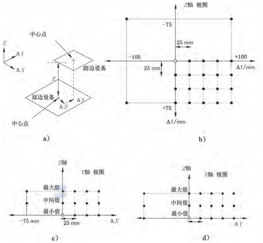
图 4 系统效率测试点分布图
