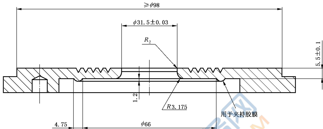
图 A.2 可选择的下夹盘
