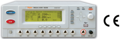
TH9201S 体积(mm): 340(W) × 120(H) × 438(D) 净重: 18.5kg
