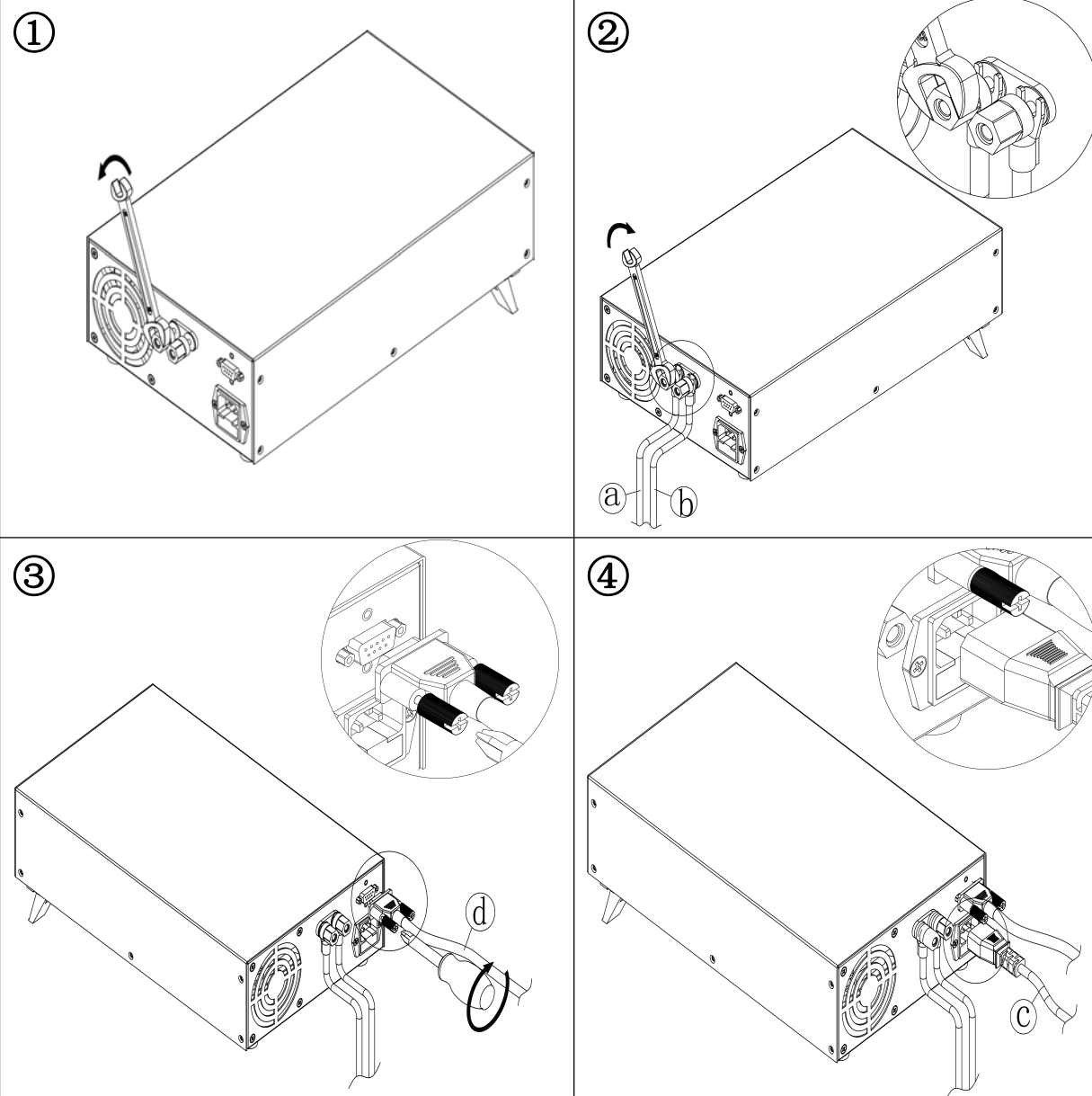
KSD-1KW系列直流电源安装示意图
