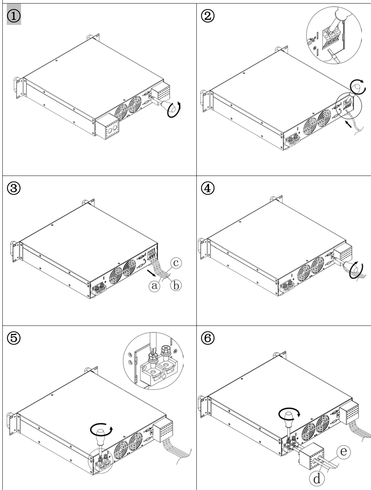
KSD-3KW系列电源安装示意图
