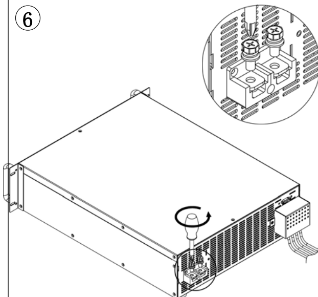
KSD-6KW/10KW 系列直流电源安装示意图
