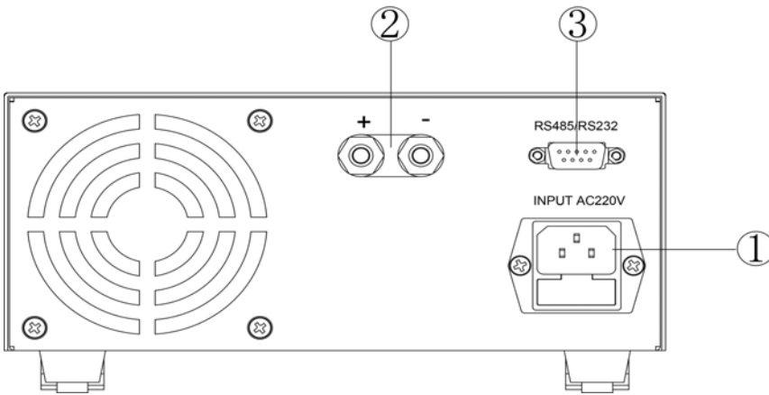
b. KSD-1KW 系列直流电源接口示意图
