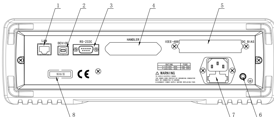
图 2-2. 后面板说明
