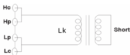
图 5—20 变压器漏感测量
