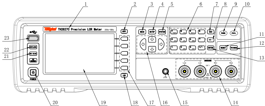
图 2-1. 前面板说明
