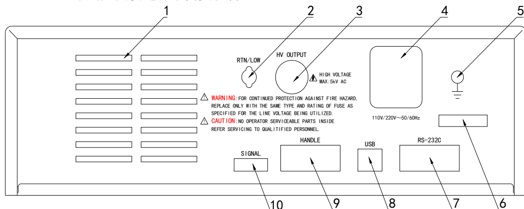
图 3-2 后面板说明
