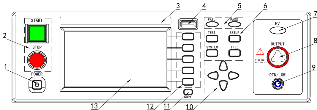
图 3-1 前面板说明
