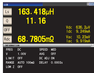
L、Q、Rdc连续测量画面
