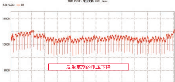
电压变动图
