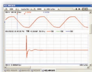
瞬态界面
