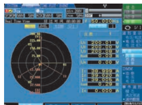
矢量图显示
