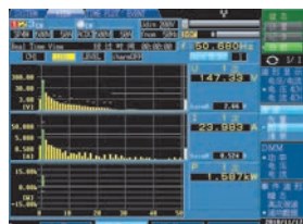
谐波图显示
