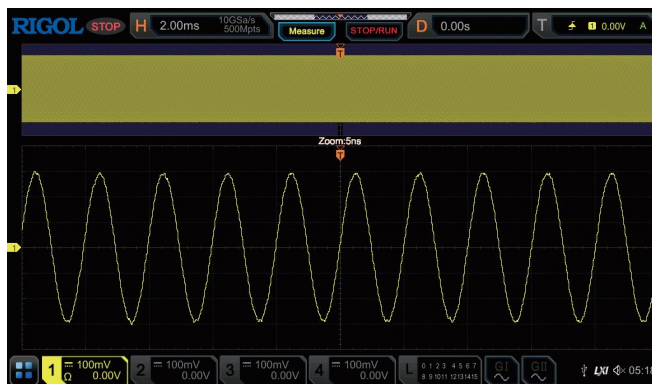
500 M 存储深度下仍保持 10 G 采样率，捕获 50 ms 时长，波形完全不失真
