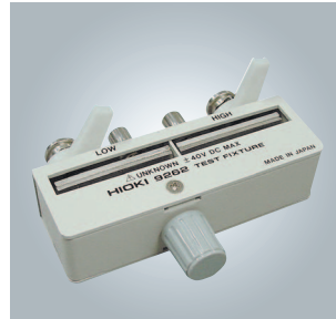
9262 测试治具
