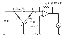
(2) 有隔离点，因 E_m \approx 0 ，故 I_r \approx 0 ，可以只对 I_x 进行测试。
