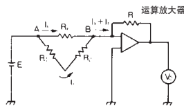
(1) 无隔离点，受周围回路的电流 I_r 的影响
