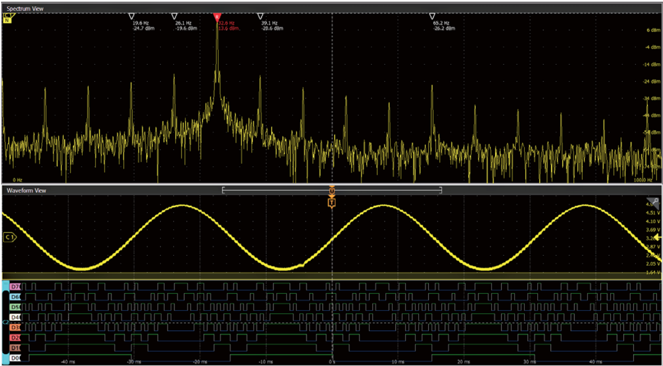
FlexChannel 输入并不只是模拟输入和数字输入，还包括频谱视图。这种泰克已获专利的技术可以同时查看所有模拟信号的模拟视图和频谱视图，且在每个域中进行独立控制。
