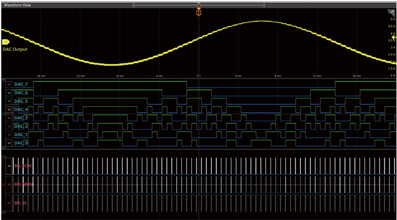
通道 2 把一只 TLP058 逻辑探头连接到 DAC 的 8 个输入上。注意绿色和蓝色颜色代码，1 为绿色，0 为蓝色。通道 3 的另一只 TLP058 逻辑探头探测驱动 DAC 的 SPI 总线。白边表示有更高频率的信息可以放大，也可以在下次采集时迁移到更快的扫描速度。
