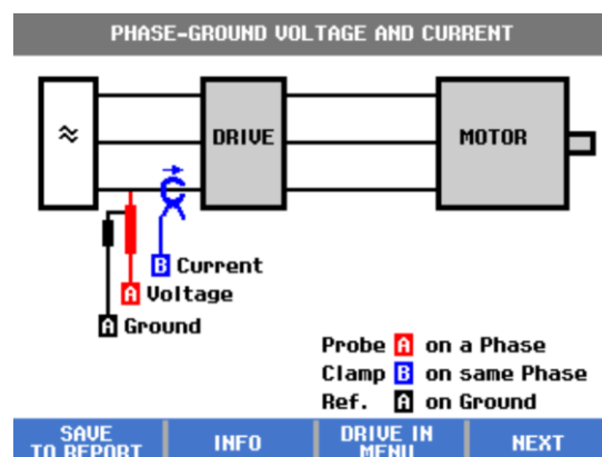
驱动输入逐步引导测量连接
