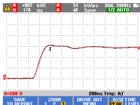
带缩放的电压调制
