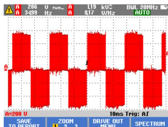
采用自动触发捕获的驱动输出波形
