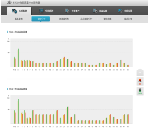
图 6 E2000web 界面一谐波柱状图
