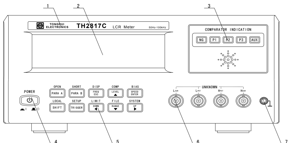
图 3—1 前面板
