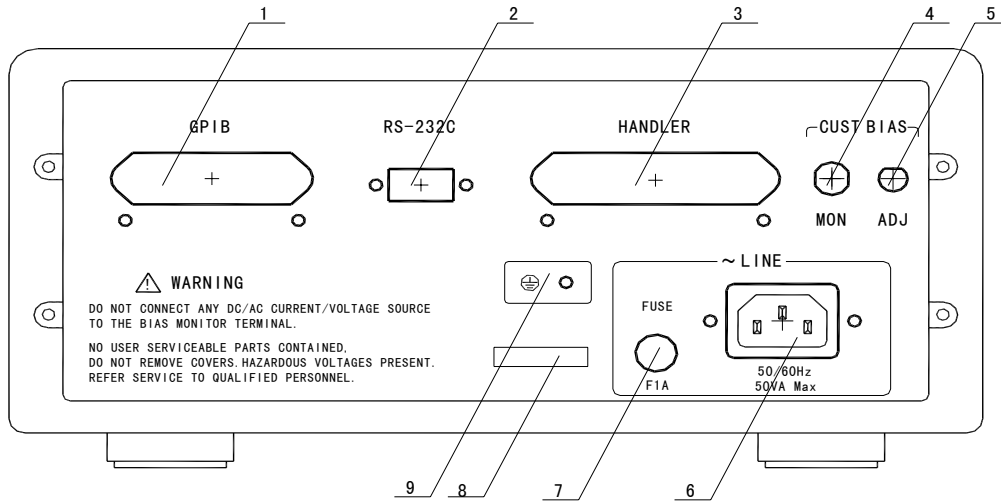
图 3—2 后面板
