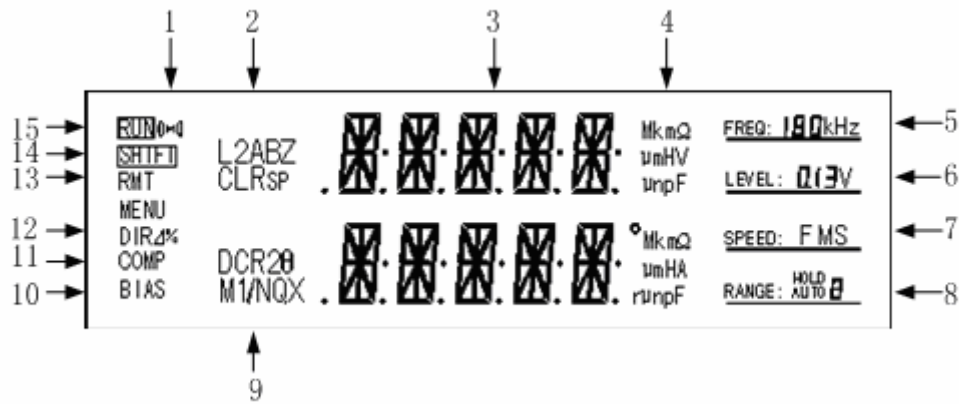
图 3—3 显示区域
