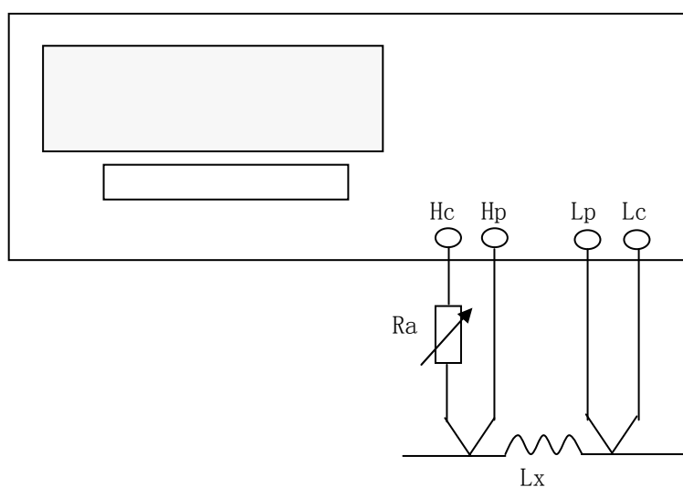
图 5—9 信号源内阻调节示意图
