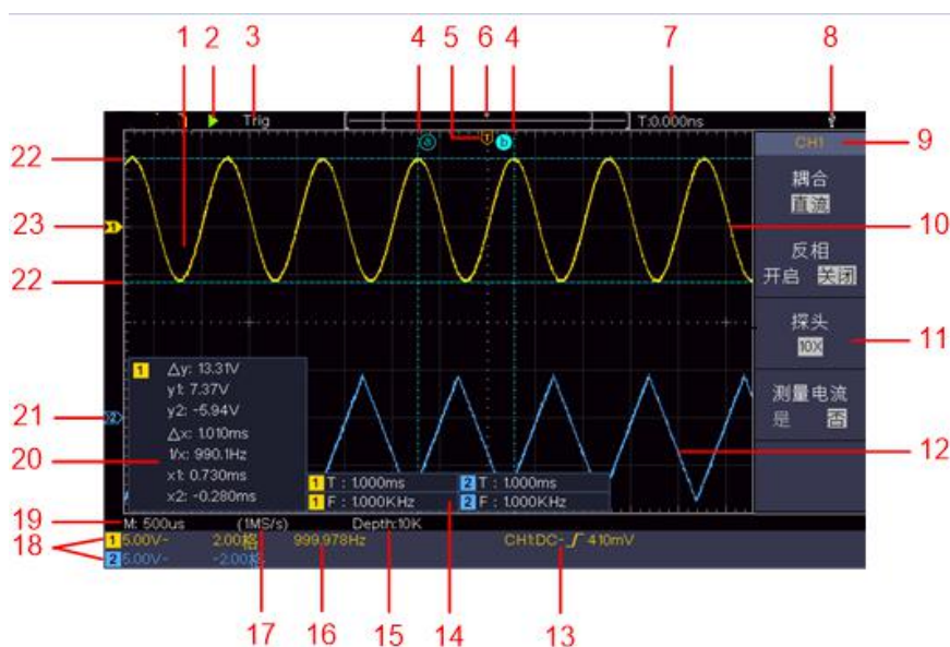
图 3- 4：显示界面说明图
