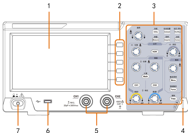
图 3- 1：示波器前面板
