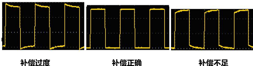
图 3- 6：探头补偿显示波形
