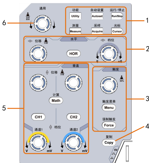
图 3- 3：按键和旋钮控制区说明图
