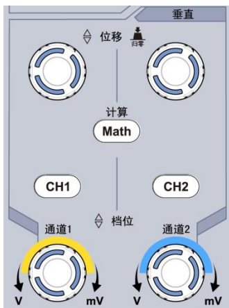
图 3- 10：垂直控制区
