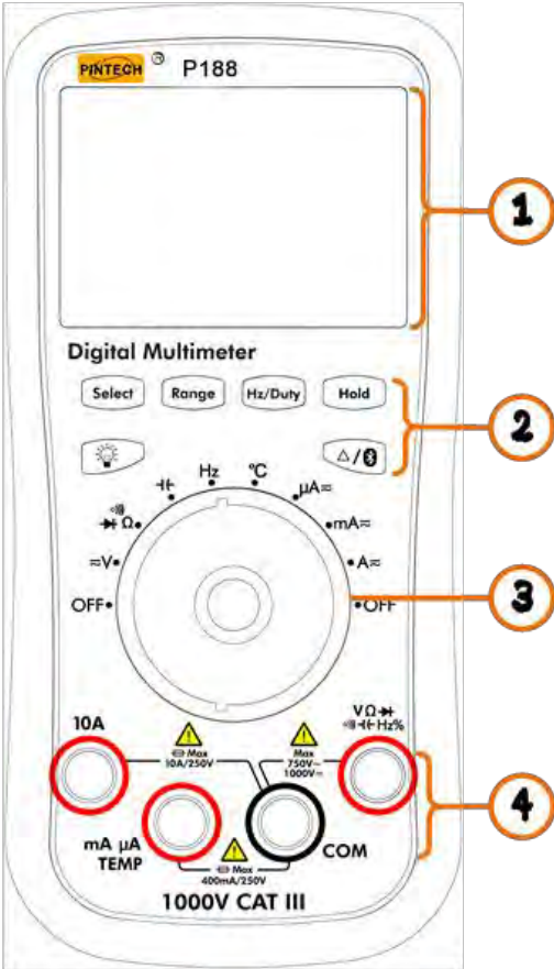
图 2-1 前面板概览
