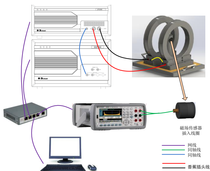
系统测试连接示意图:
