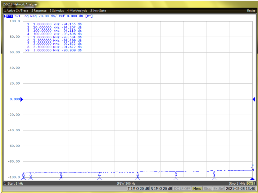
CM 03203M 宽带电流监测钳 s21 曲线*
