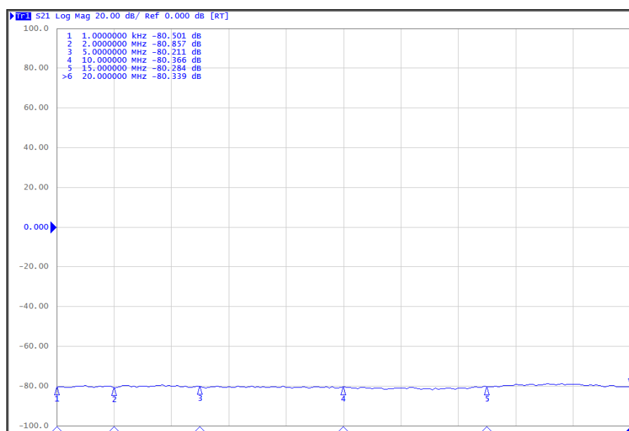
CM 0220M 宽带电流监测钳 s21 曲线*
