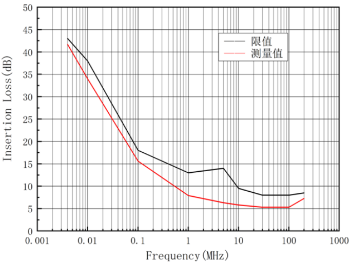
BCIP-200 电流注入钳插入损耗曲线
