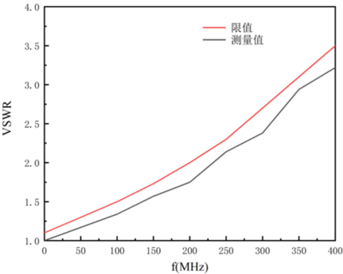
BCICF-400 电流耦合钳校准夹具电压驻波比曲线
