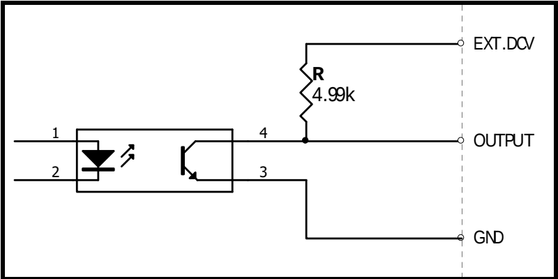
图 8-3 输出端原理图 (分选, IDX, EOM)
