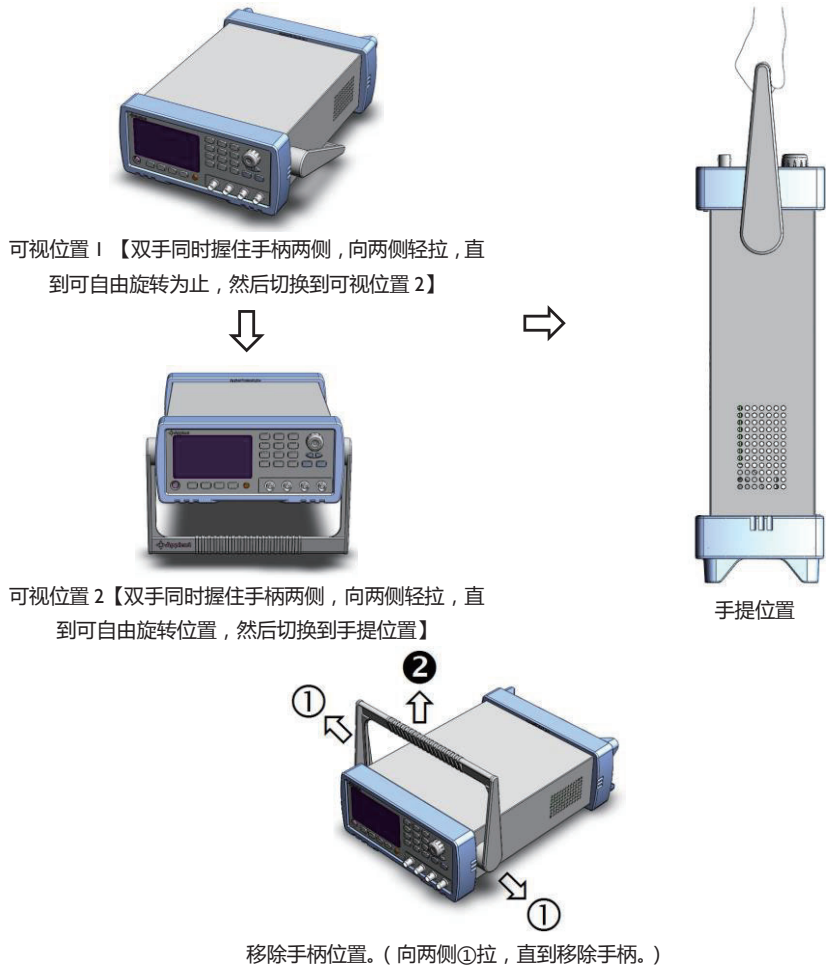
图 1-2 仪器手柄(示意图,面板图形与实际不符)
