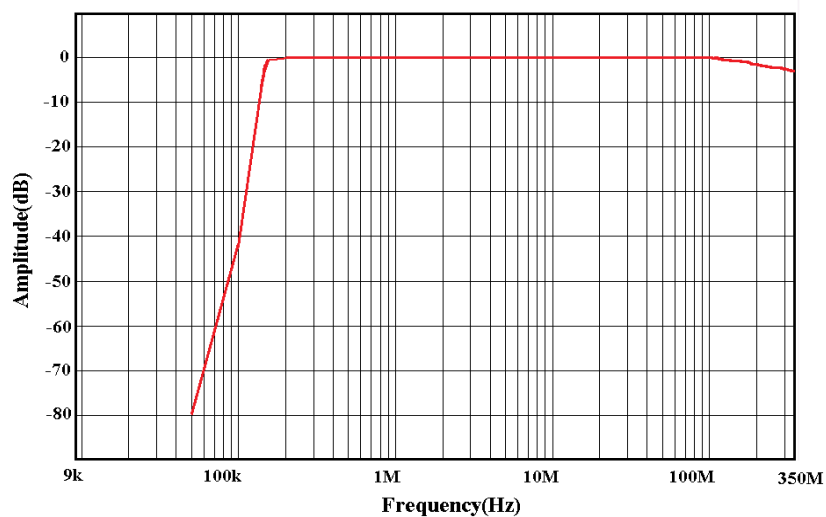
图 1 频响曲线
