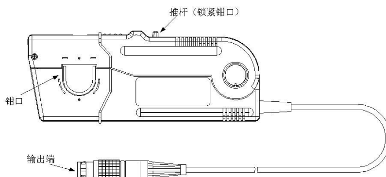
图 4: CP3030 和 CP4040 结构图
