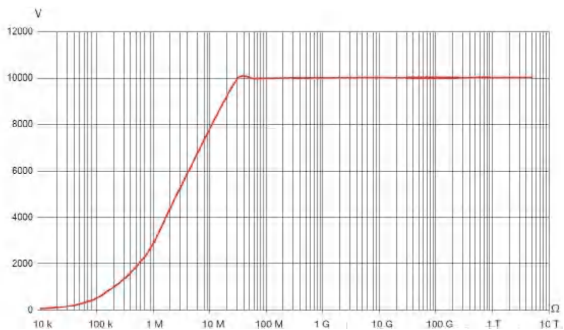
10000V 量程
