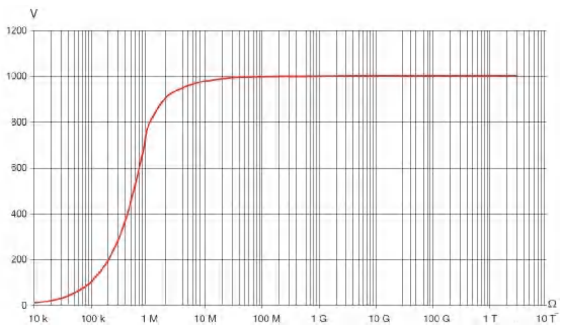
1000V 量程
