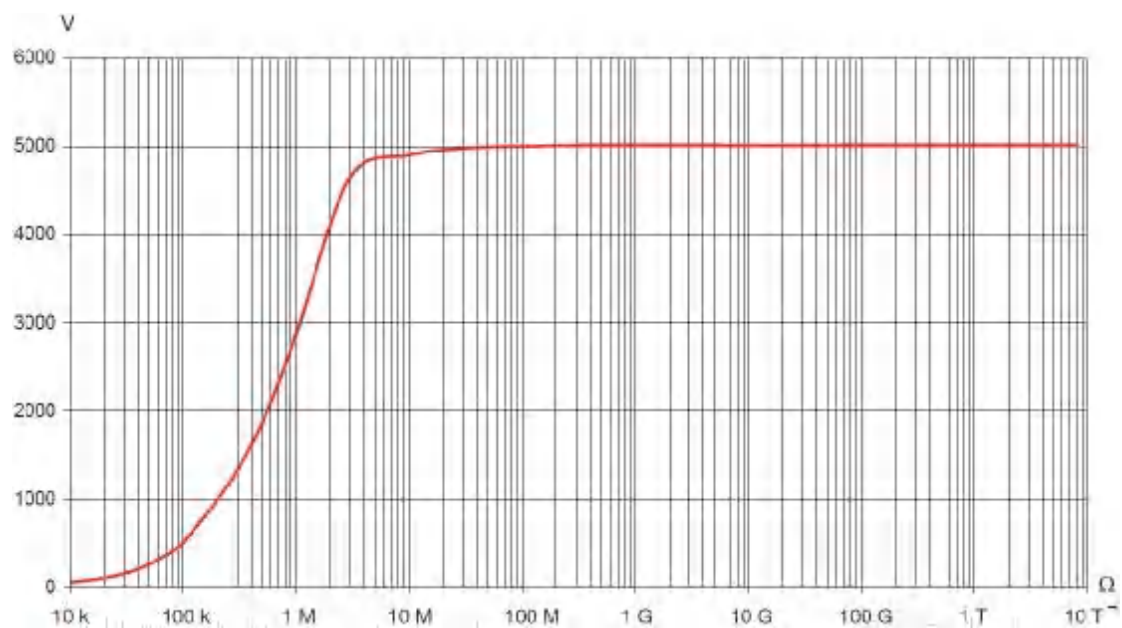
5000V 量程
