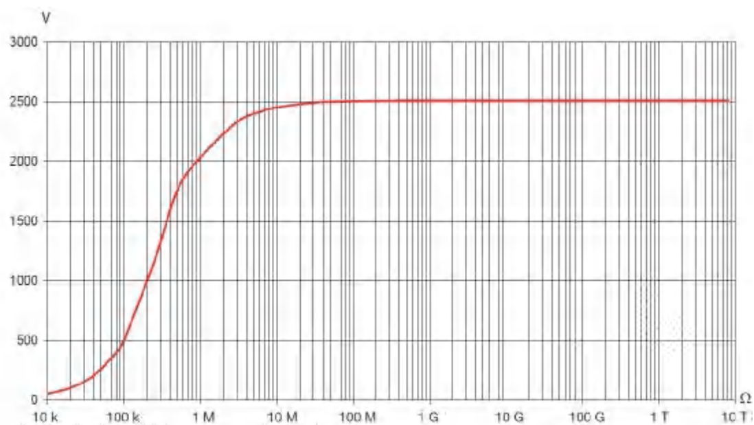
2500V 量程
