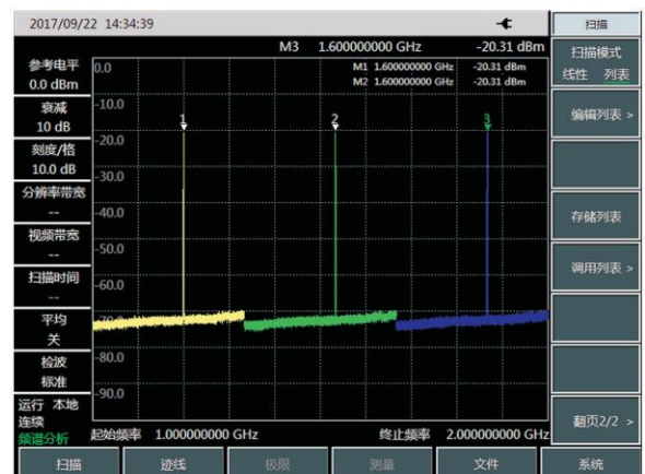
列表扫描
