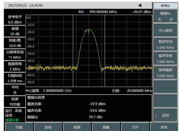
载噪比
