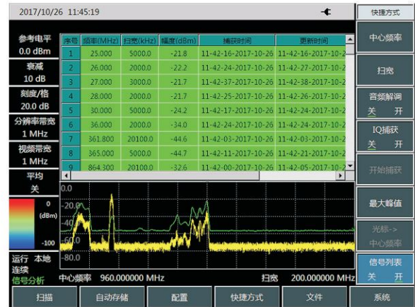
信号分析
