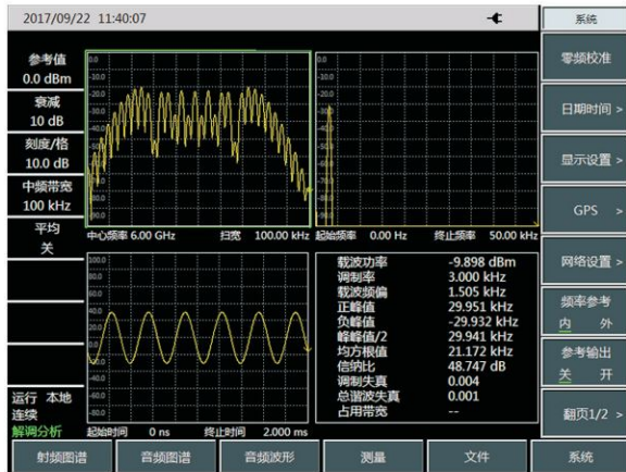
模拟调制
