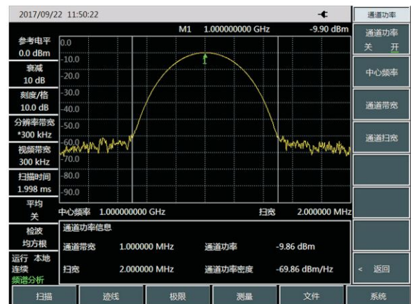
通道功率
