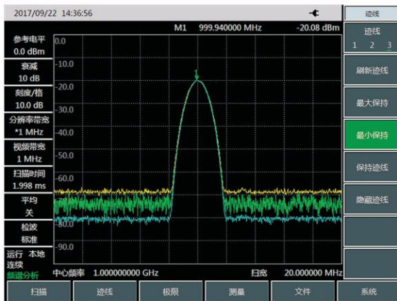
多迹线
