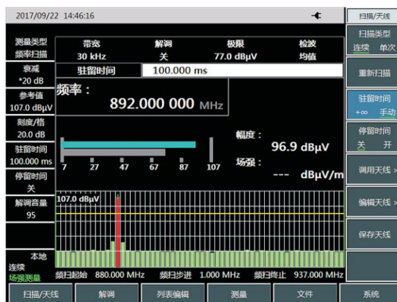
场强测量
