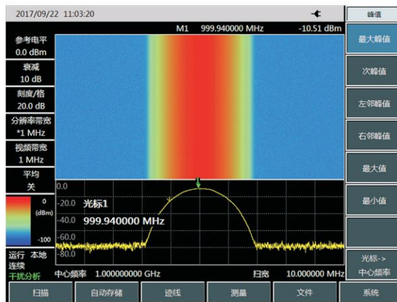
干扰分析（瀑布图）
