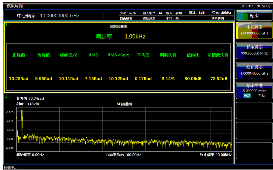
图 4.25 \Phi M 信号基带频谱图
