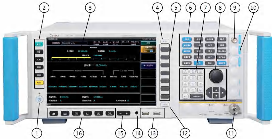
图 3.12 3927 前面板
