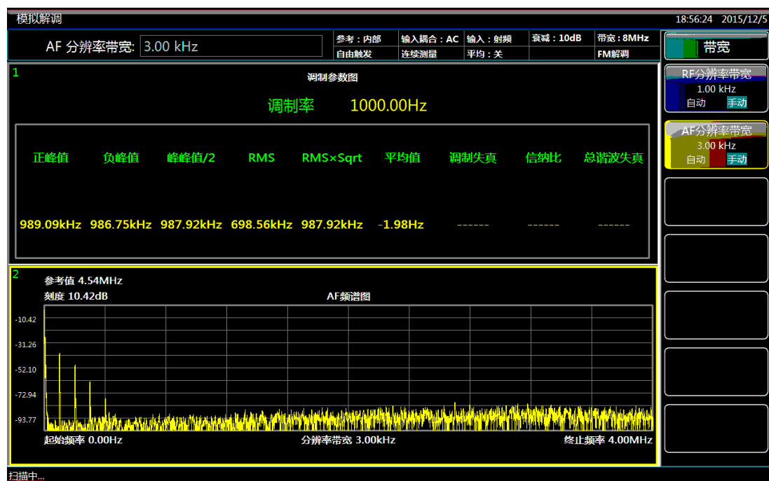
图 4.21 FM 信号基带频谱图
