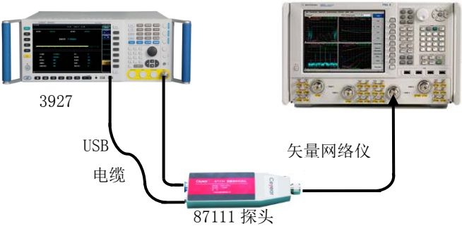
图8.7 电压驻波比测试示意图
