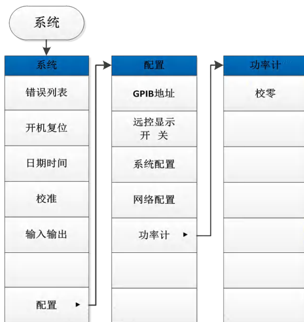
图 5.1-15 系统菜单
