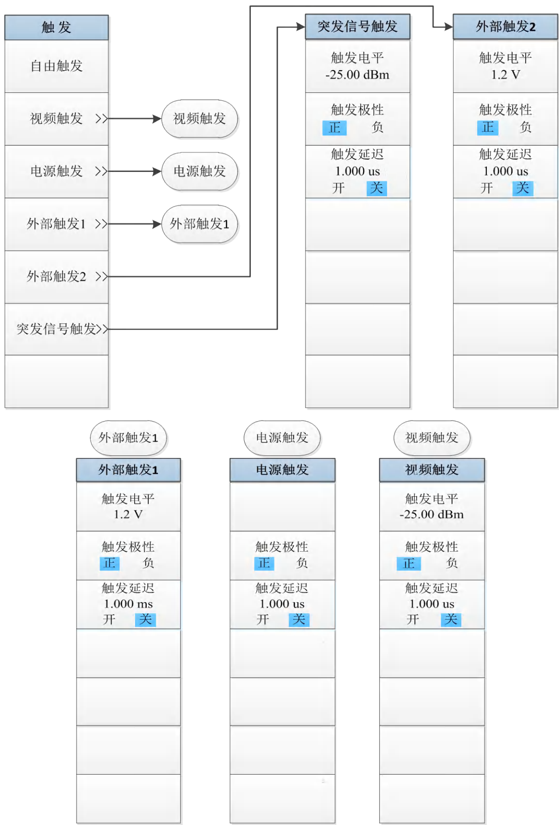
图 5.1-21 触发菜单
