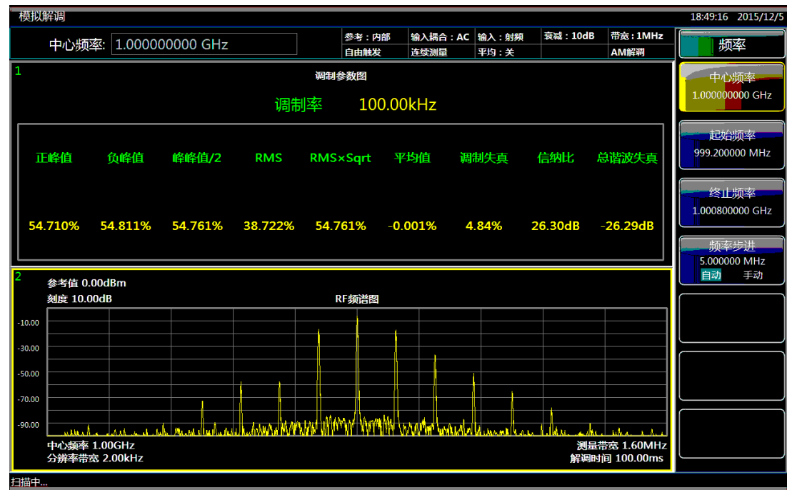
图 4.16 AM 信号射频频谱图
