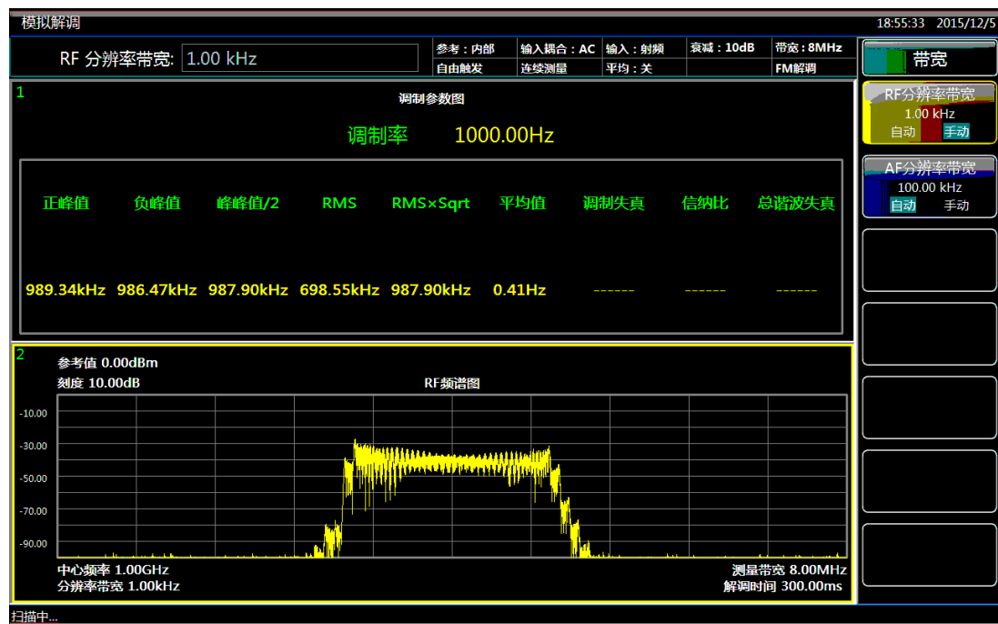
图 4.20 FM 信号射频频谱图
