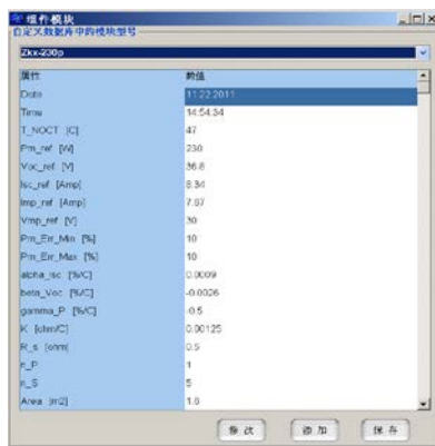
图 B-6 组件模块型号及其参数列表
