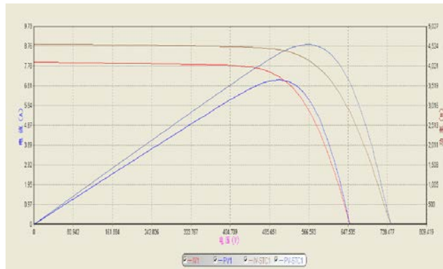
图 B-2 曲线显示窗口示意图
