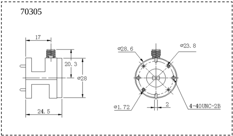
70305 结构尺寸（mm）
