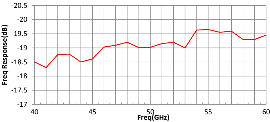
检波频响 VS 频率
