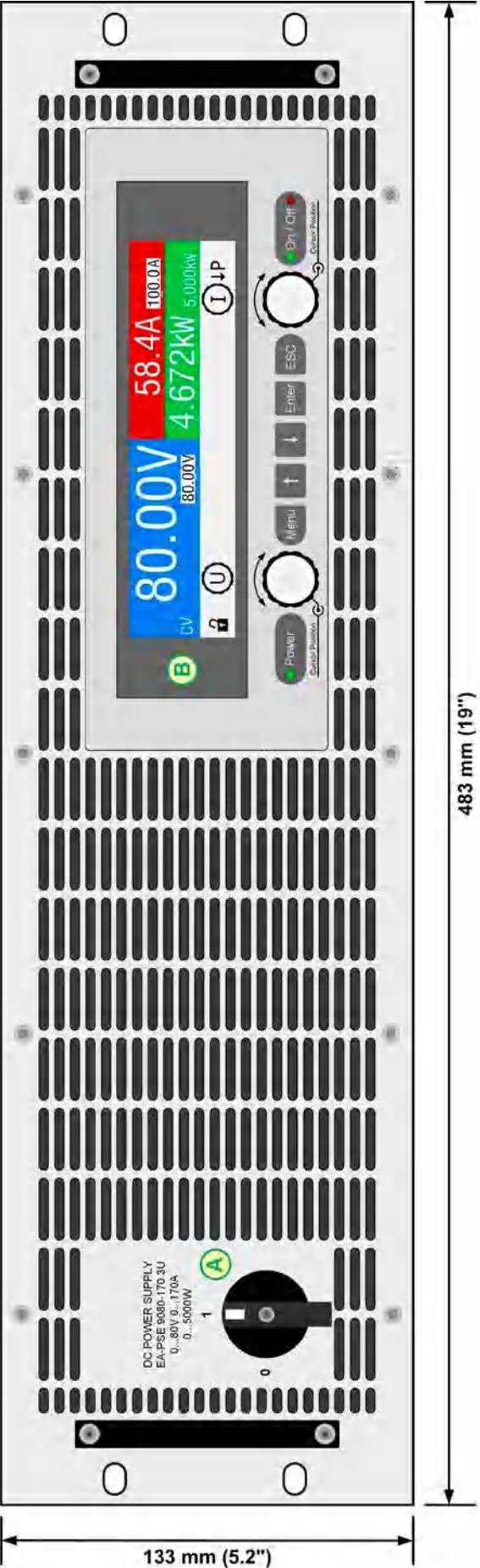
图 1 - 前视图
