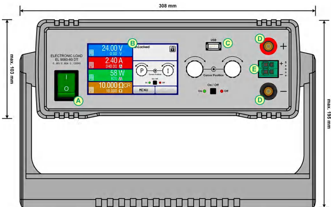
图 1 - 前视图
