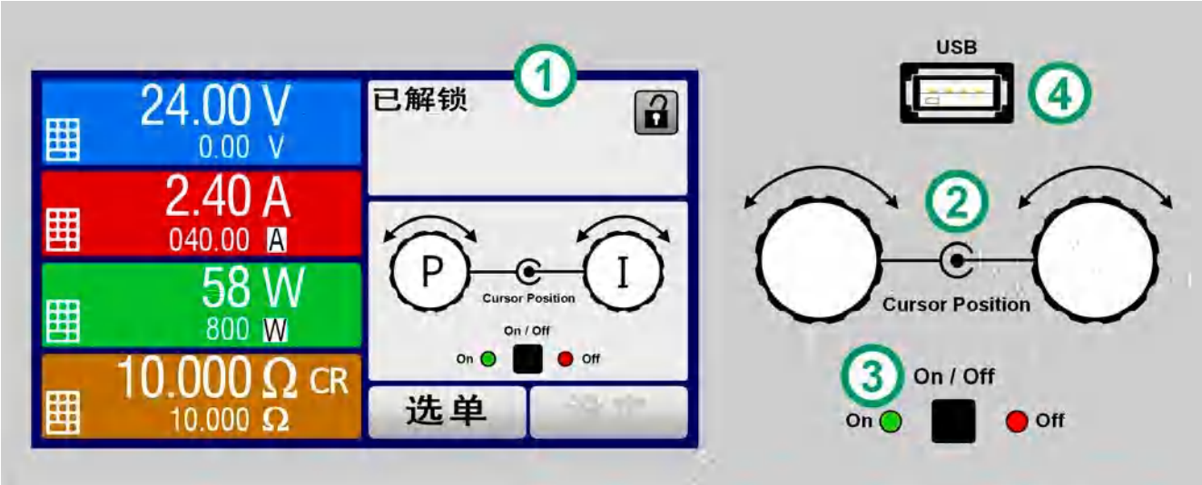
图 5 - 控制面板
