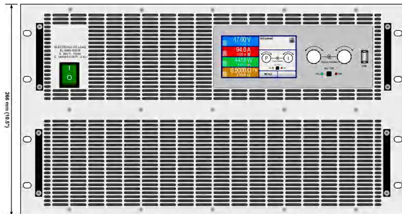
图 6 - 前视图
