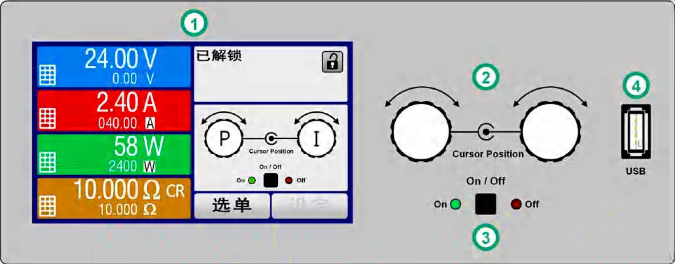
图 11 – 控制面板
