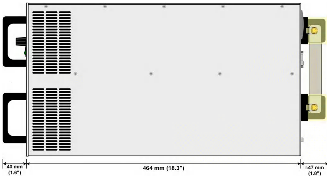
图 8 - 侧视图，装有直流端子盖（针对500 V或750 V额定电压的型号）
