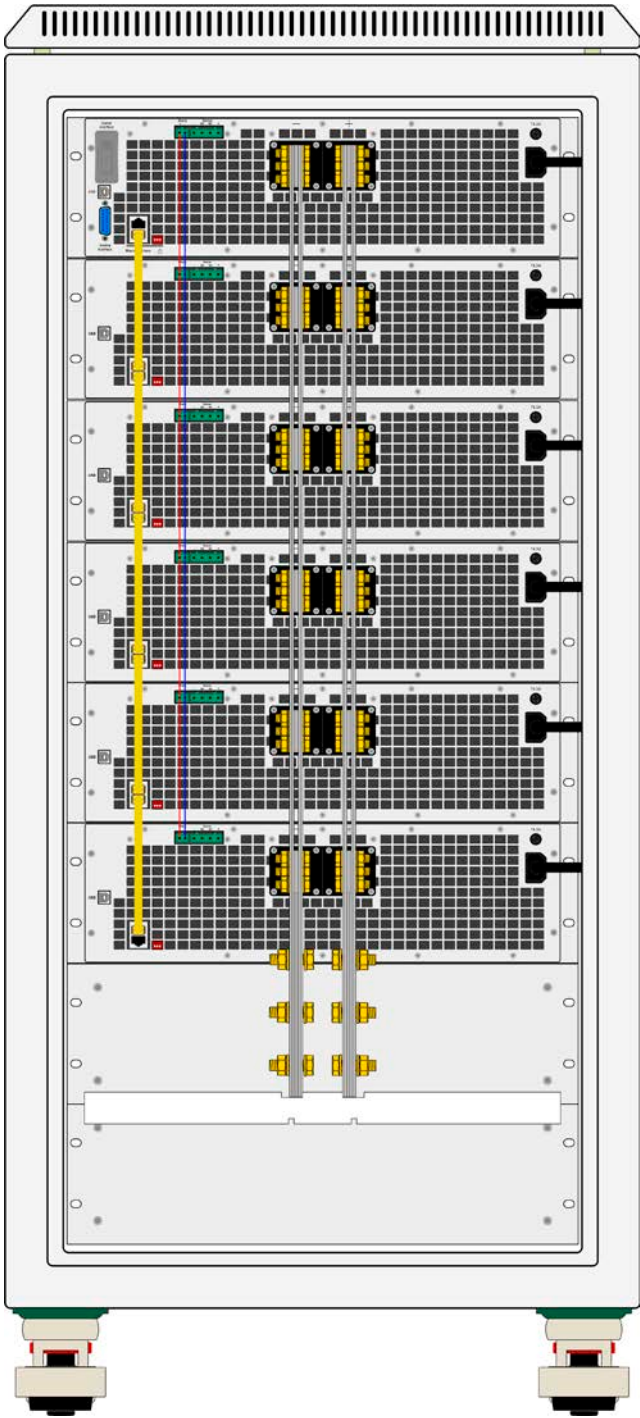
图 4 - 后视图（24U机柜范例）
