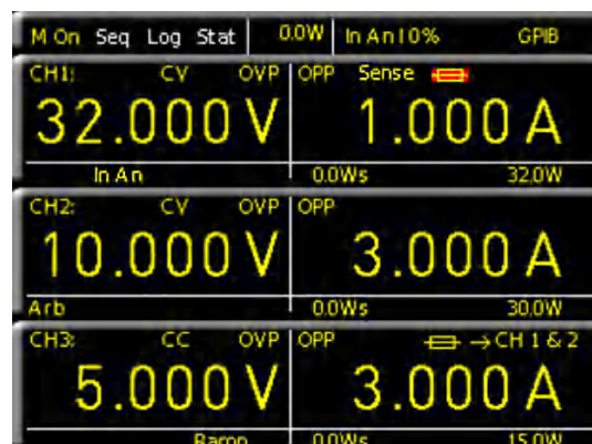
Abb. 4.3: Messwertanzeige R&S®HMC8043
