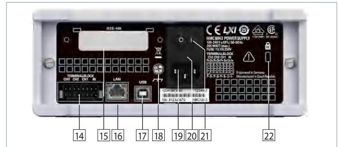
Abb. 2.2: Geräterückseite R&S®HMC8043
