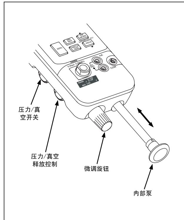
图 3. 泵特性
