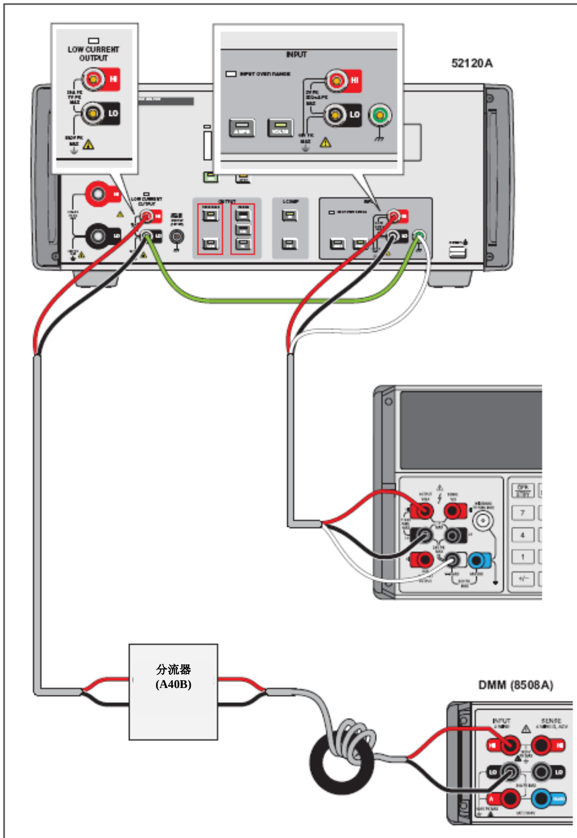
图 2-1. 降低共模干扰的连接方法
