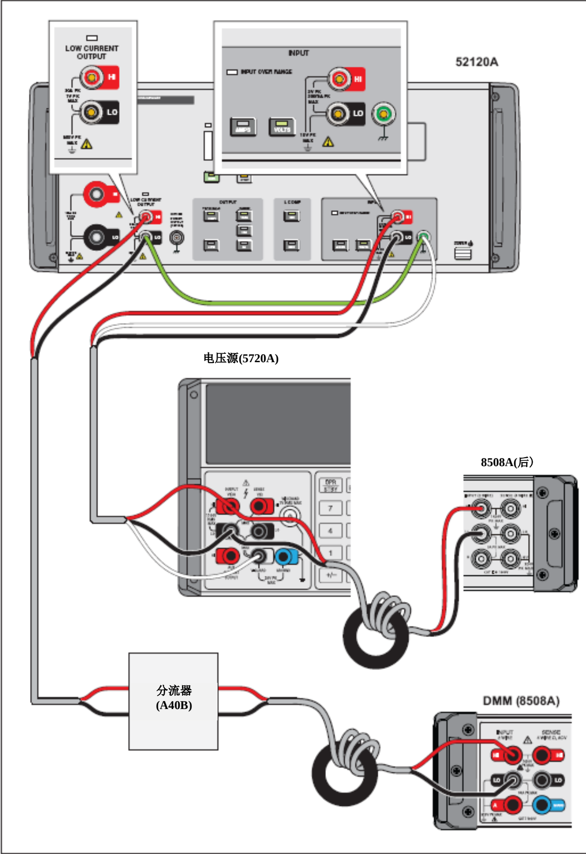
图 5-1. 测试设备连接
