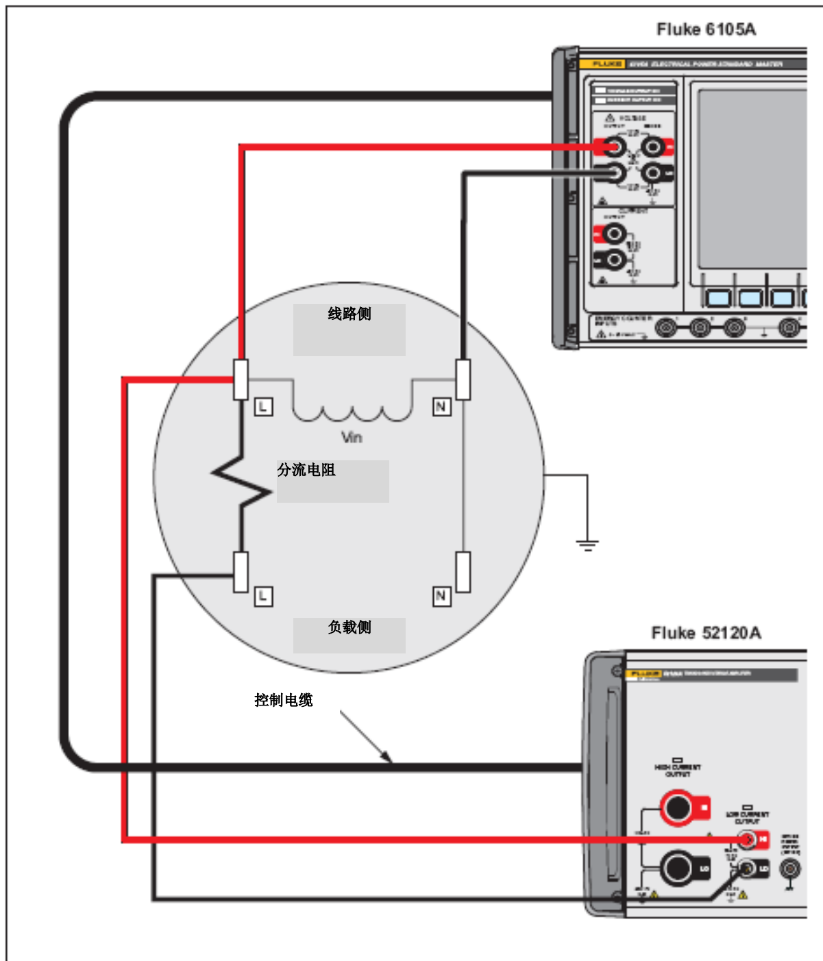
图 2-2. 仪器连接至瓦时表的方法
