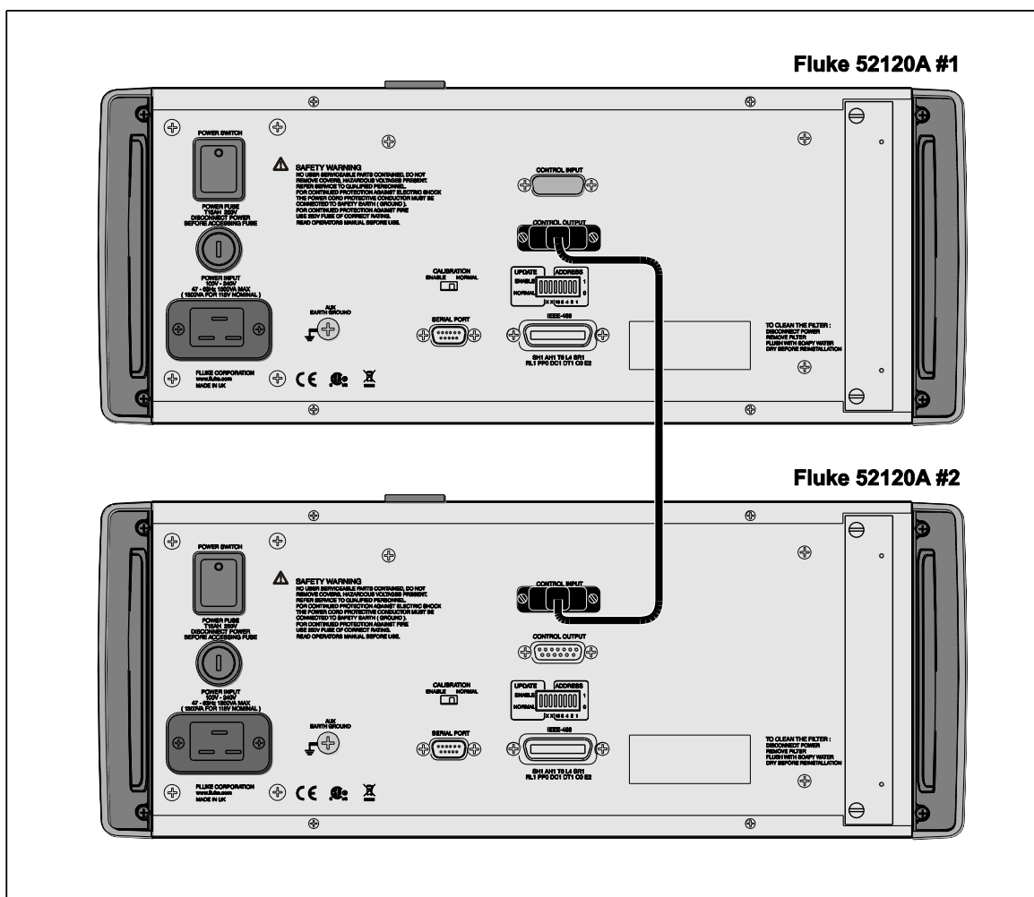
图 2-5. 主控制器到从机的连接
