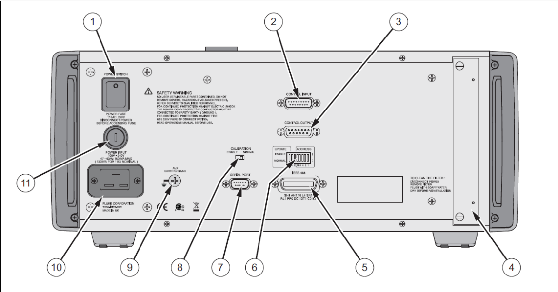
图 1-2. 后面板视图
