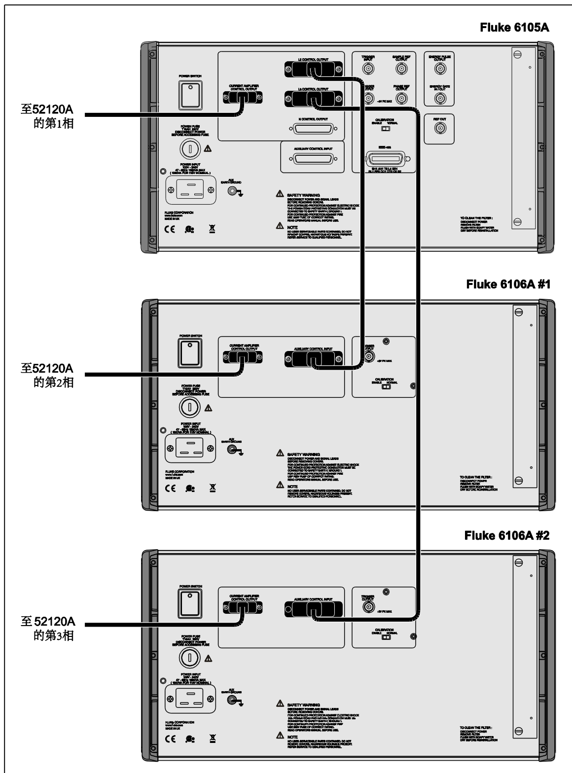
图 2-9. 6105A 和 6106A 的连接
