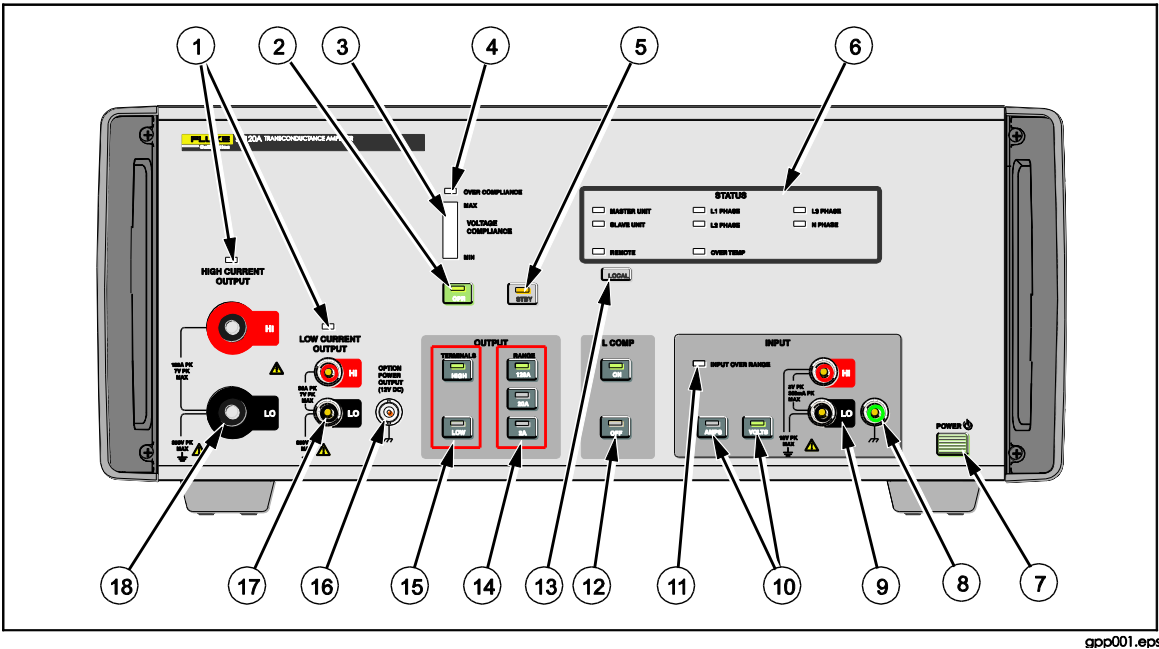
图 1-1. 前面板视图
