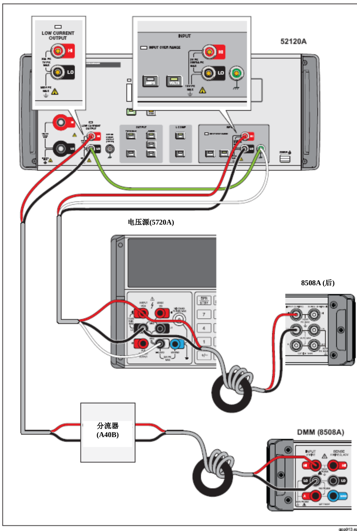
图 5-2. 校准调整步骤
