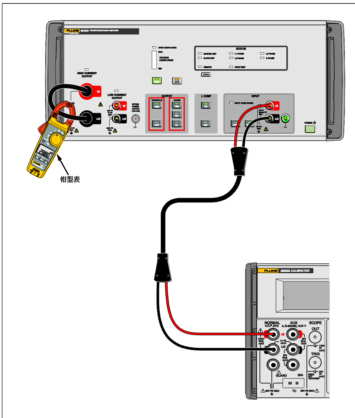
图 2-4. 5520A 和 52120A 的连接
