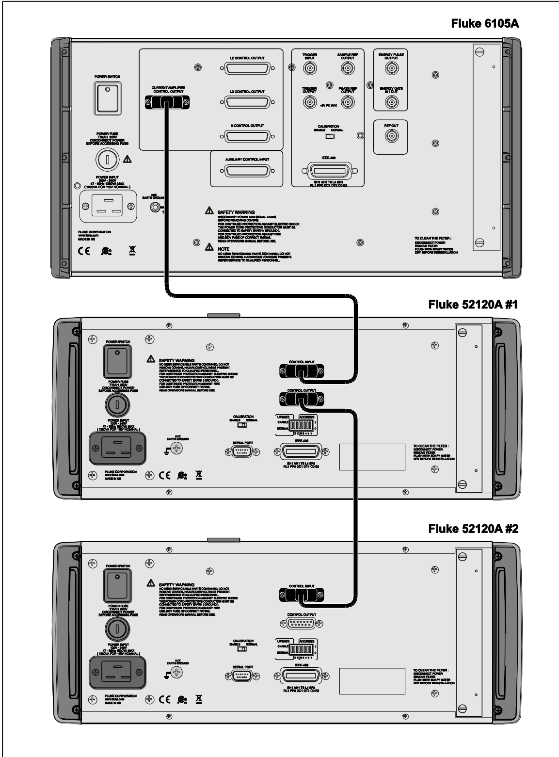
图 2-8. 多台放大器连接
