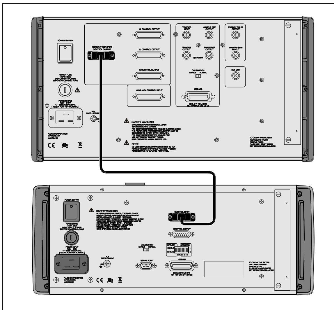
图 2-7. 反馈电缆连接
