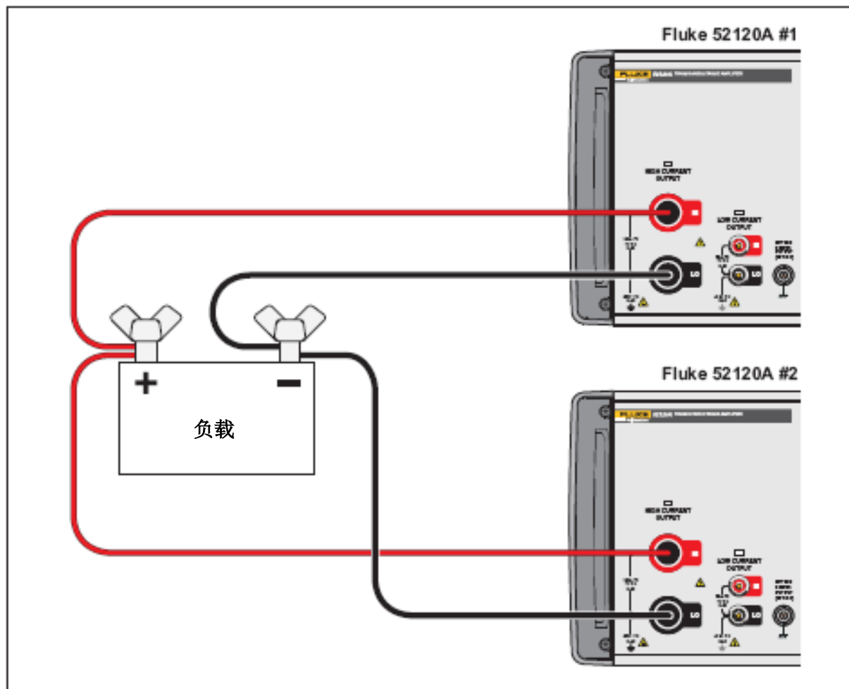
图 2-6. 两路放大器输出并联
