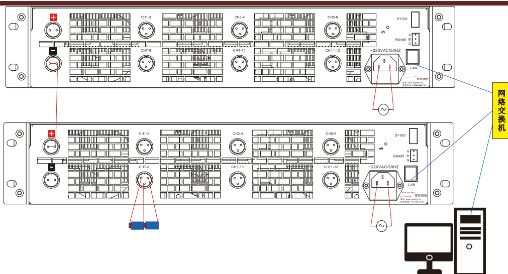
图 3-9 接线图
