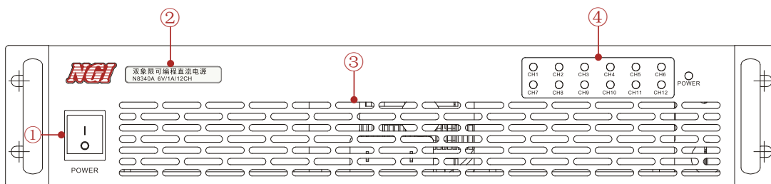
图 3-4 前面板介绍
