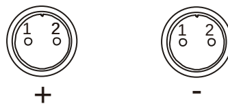
图 3-8 机箱与机箱串联正、负极
