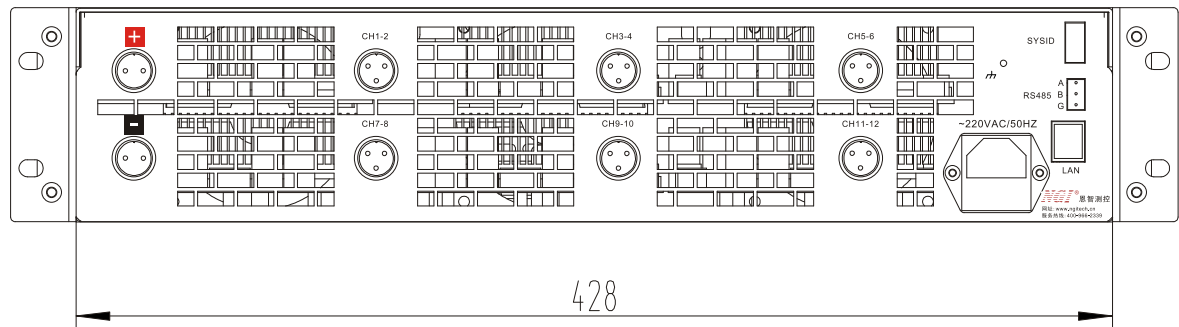
图 3-3 后面板尺寸 (mm)
