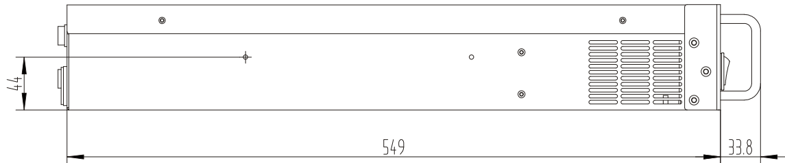
图 3-2 机箱侧视尺寸 (mm)
