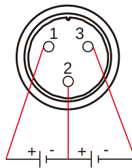
图 3-7 接线端子
