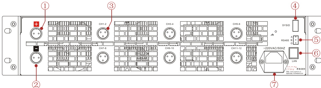
图 3-5 后面板说明
