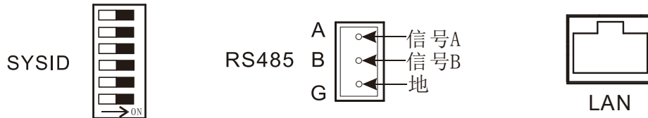
图 3-6 控制端子
