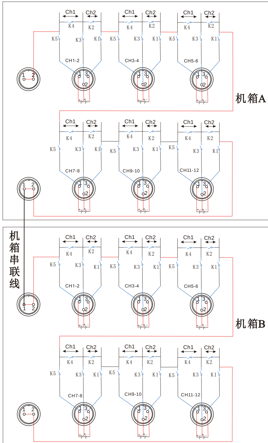
图 3-10 内部电器结构
