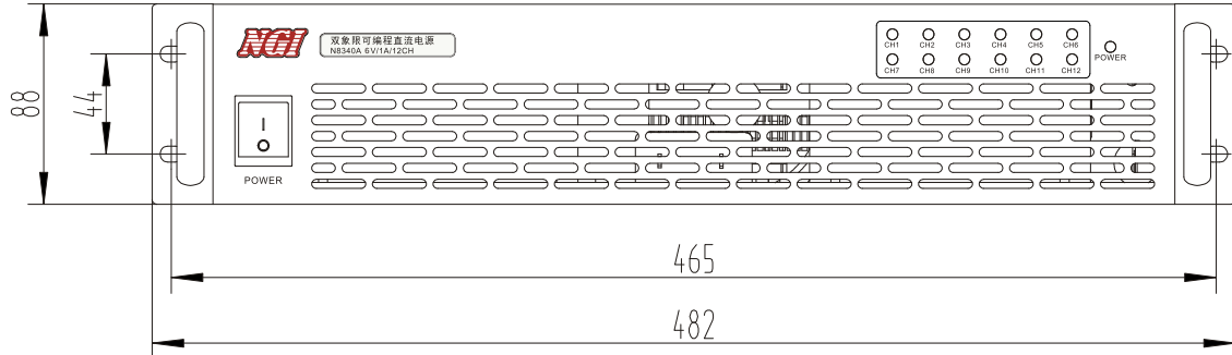
图 3-1 前面板尺寸 (mm)
