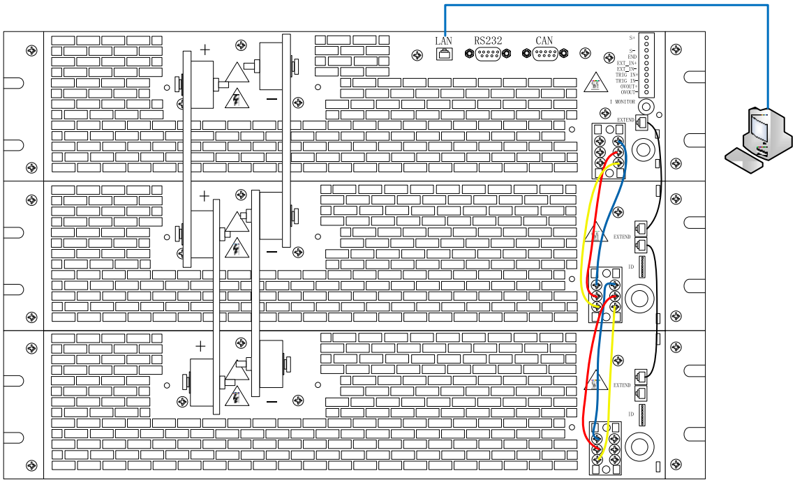
图 3-9 多机并联图
