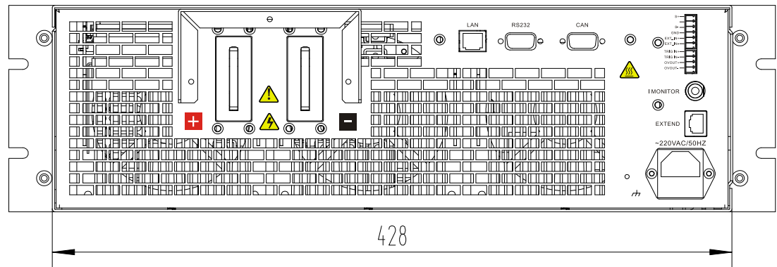
图 3-3 主机后面板尺寸图（mm）
