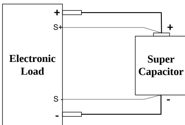
图 6-17 电容内阻测试连线图
