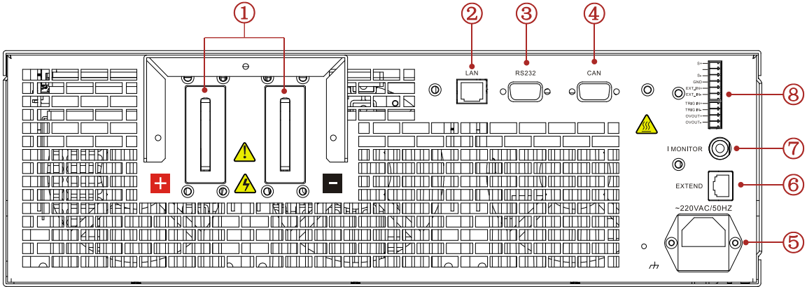
图 3-5 主机后面板
