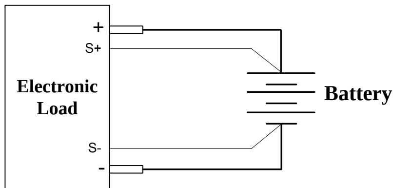
图 6-16 电池内阻测试连线图
