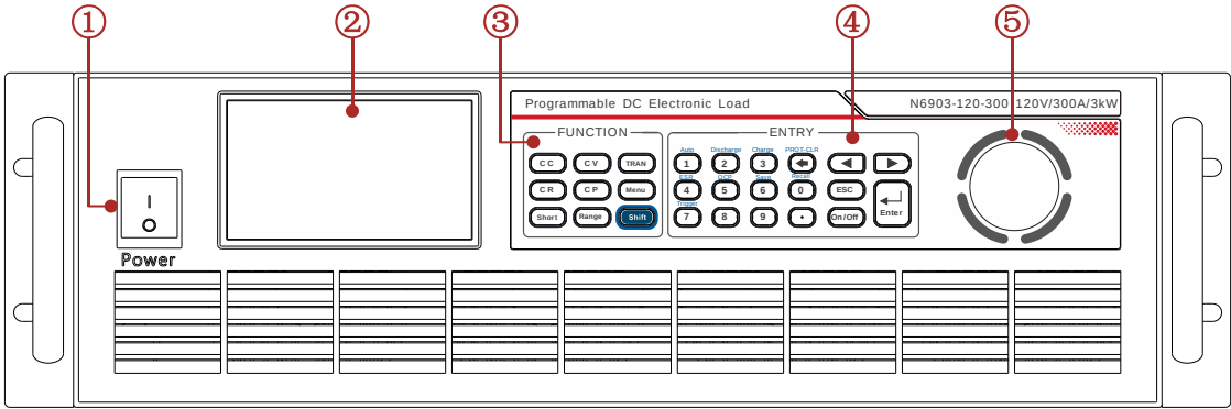
图 3-4 主机前面板
