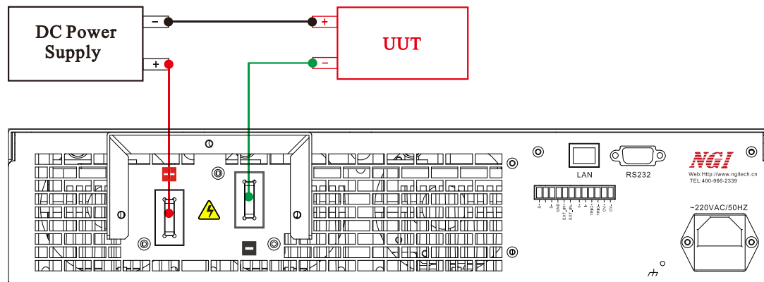
图 3-10 低电压操作
