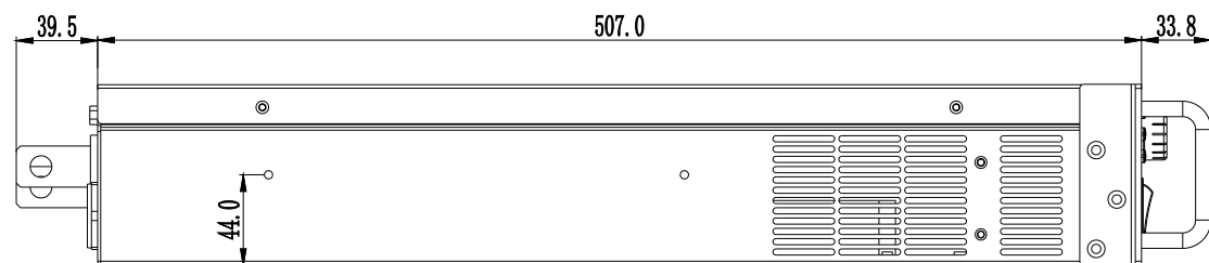
图 3-3 侧视尺寸
