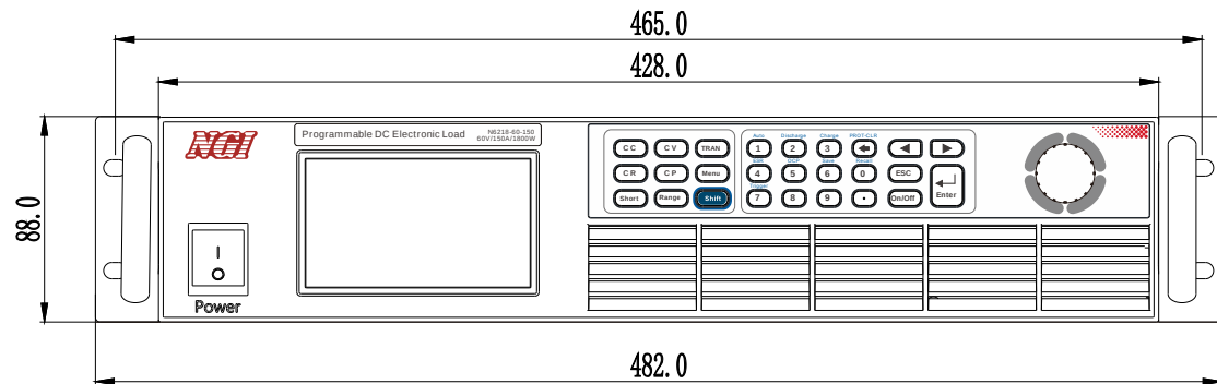
图 3-2 前面板尺寸
