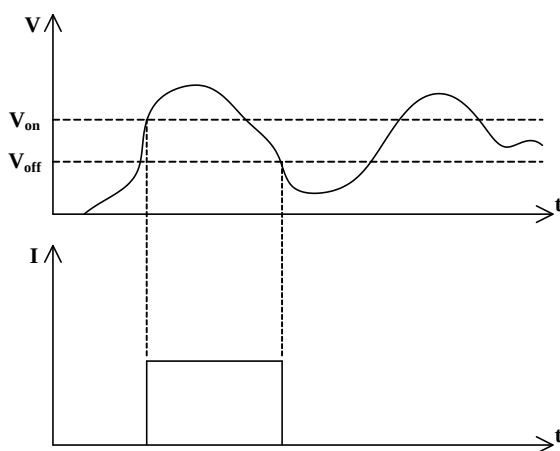
图 4-12 锁定 V_{on} 带载和 V_{off} 卸载
