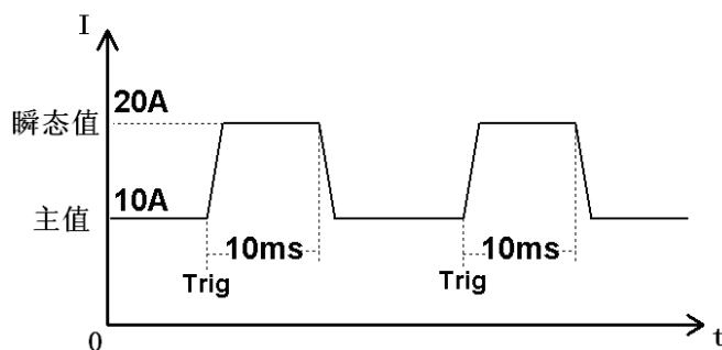
图 4-6 脉冲方式
