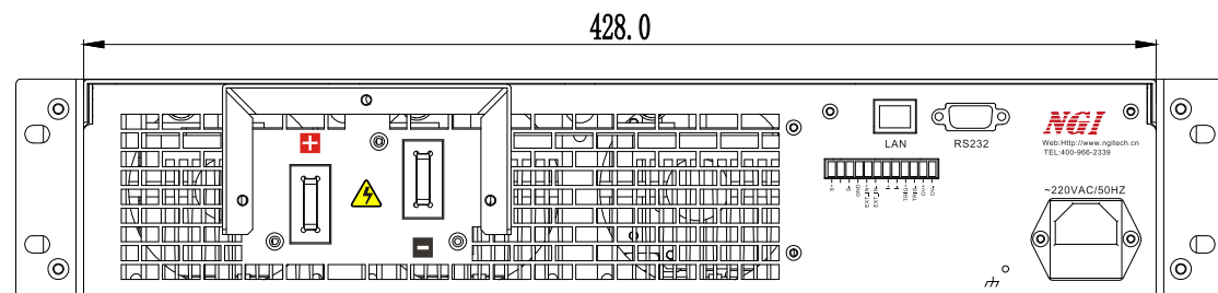
图 3-4 后面板尺寸
