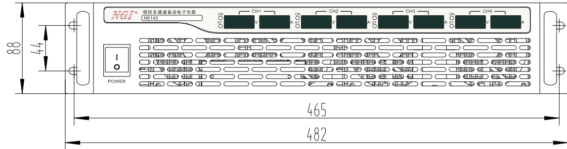
图 3-1 前面板尺寸
