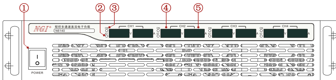
图 3-7 前面板
