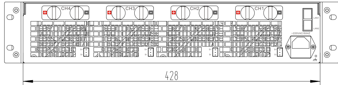
图 3-3 后面板尺寸
