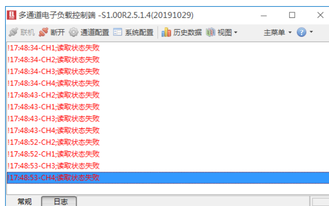
图 4-20 日志
