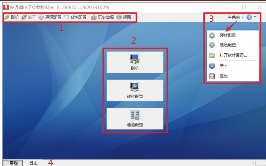
图 4-19 程序主界面
