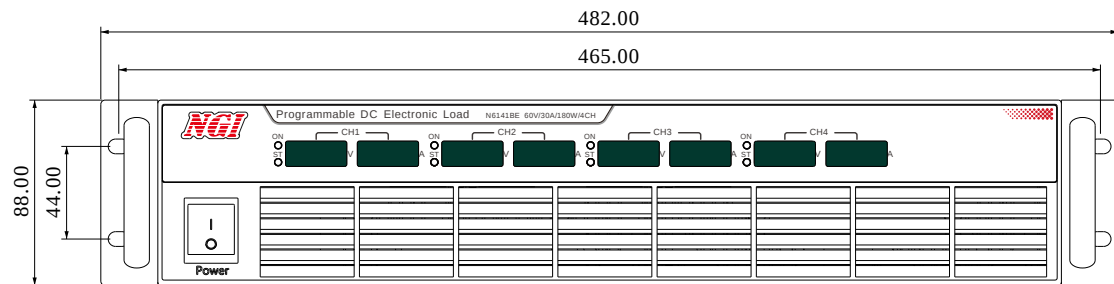
图 3-4 前面板尺寸
