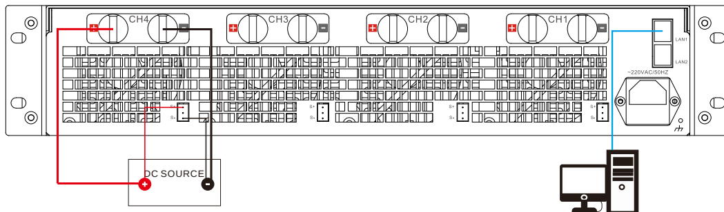
图 3-9 设备接线图
