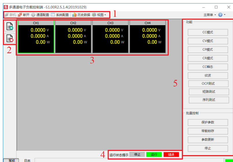
图 5-1 联机主界面
