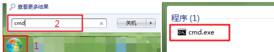
图 4-11 打开 cmd
