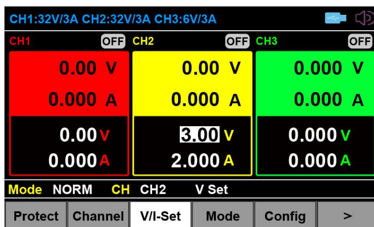
图 3-3 设置电压/电流
