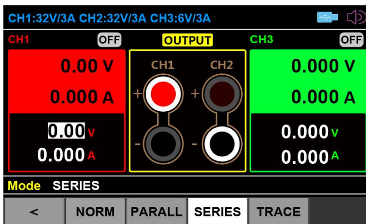
图 3-9 串联模式
