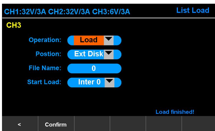
图 3-17 序列下载
