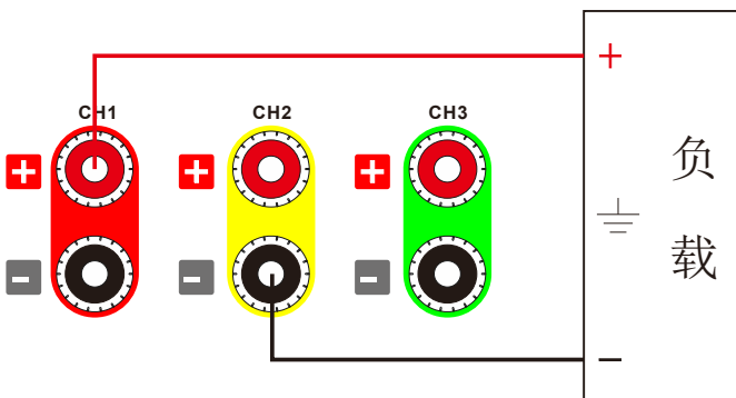
图 3-10 串联模式接线
