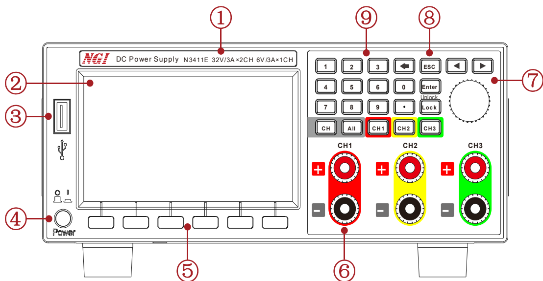
图 2-5 N3410 前面板
