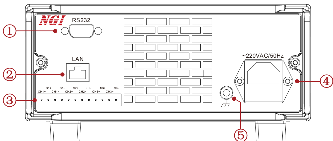
图 2-6 N3410 后面板
