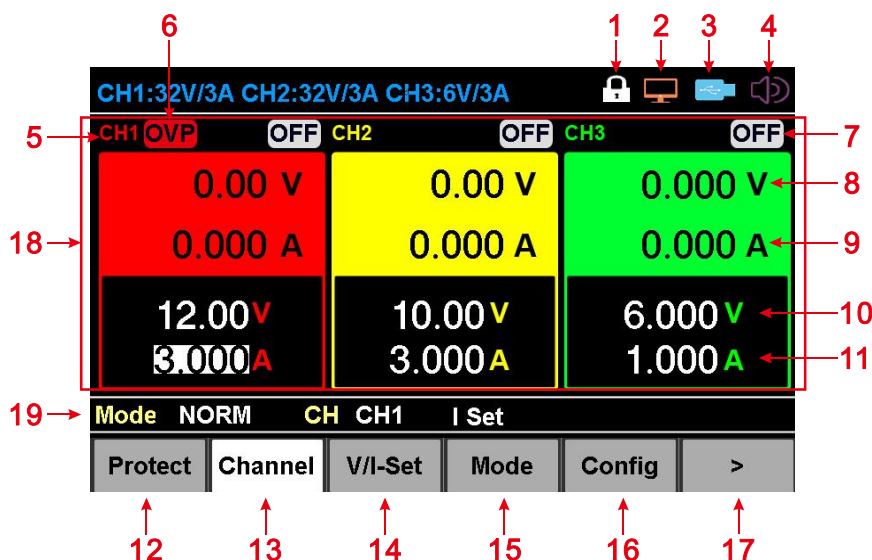
图 3-1 主界面
