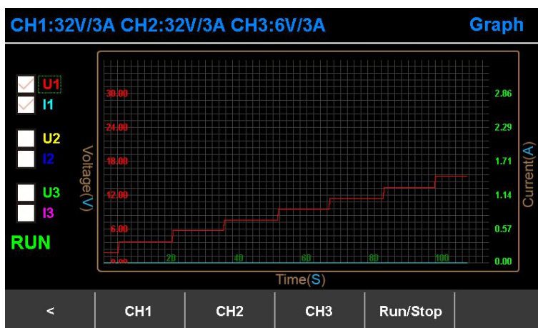
图 3-18 图形显示
