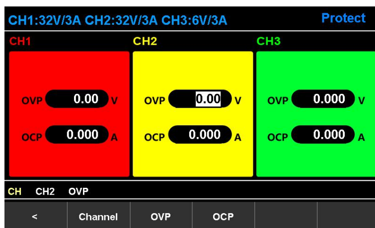
图 3-4 保护设置
