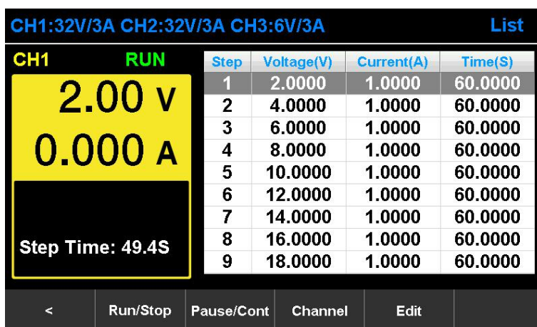
图 3-15 序列模式
