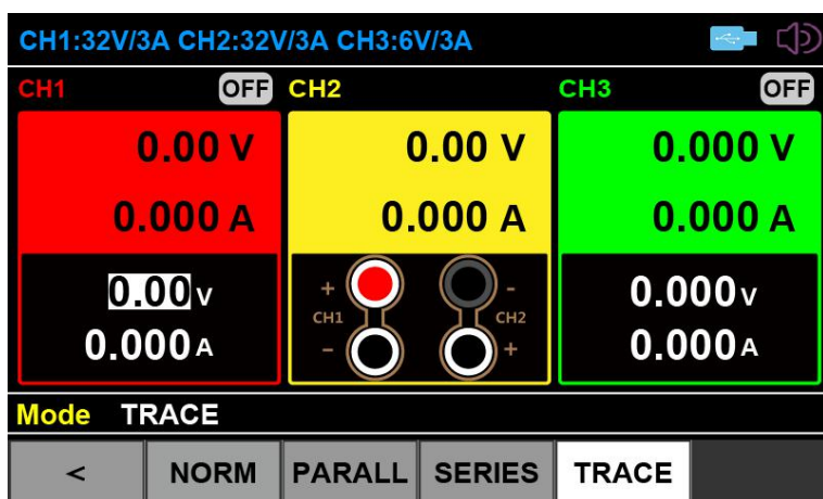
图 3-11 跟踪模式
